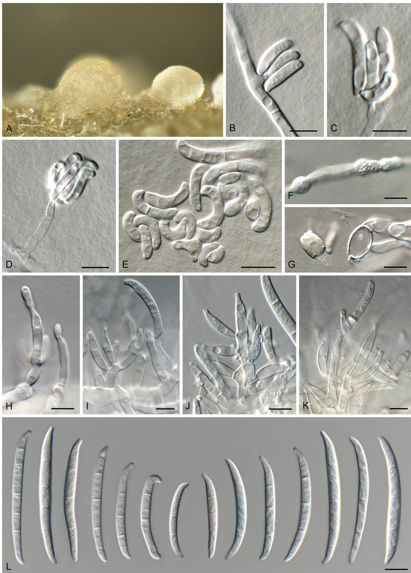
Fig. 7. Fusarium algeriense (CBS 142638). A. Sporodochium on CLA. B–D. Aerial conidiophores with monophialides. E. Microconidia. F, G. Chlamydospores. H–K. Sporodochial conidiophores. L. Macroconidia. Scale bars = 10 µm.
