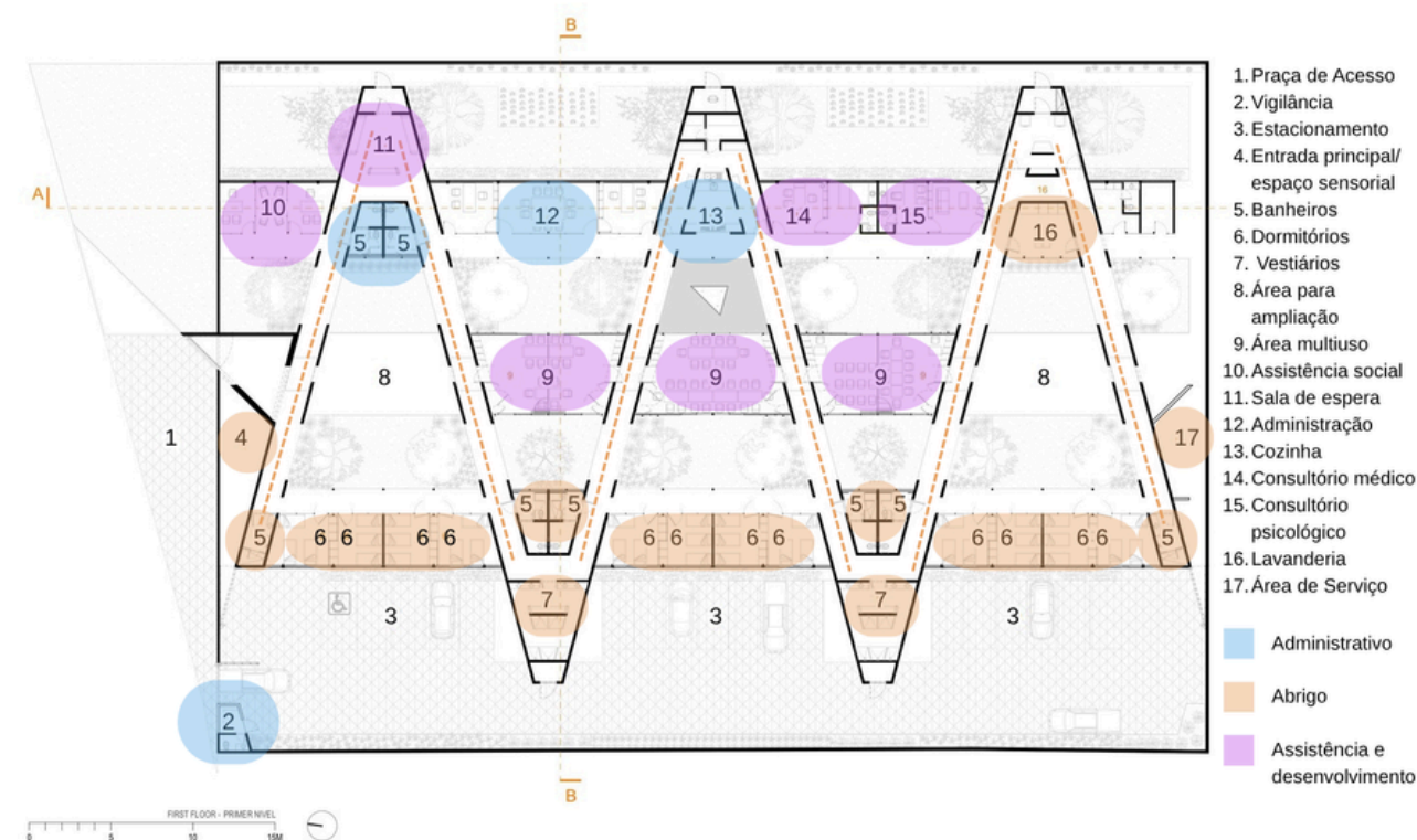
Planta Baixa do edifício.
