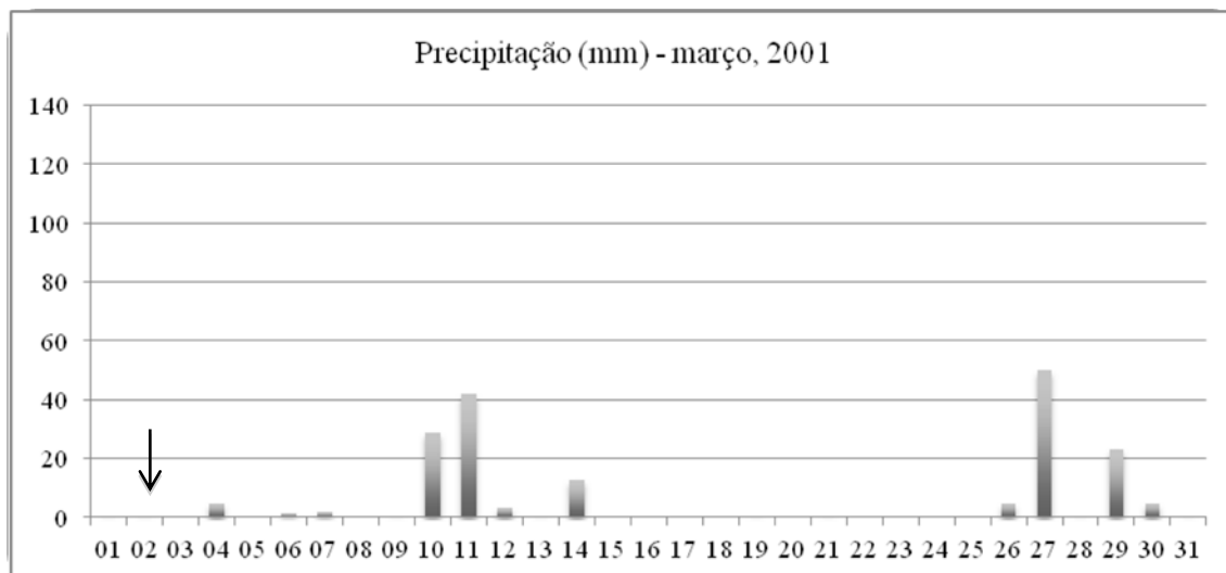
Gráfico 7 – precipitação em março de 2001
