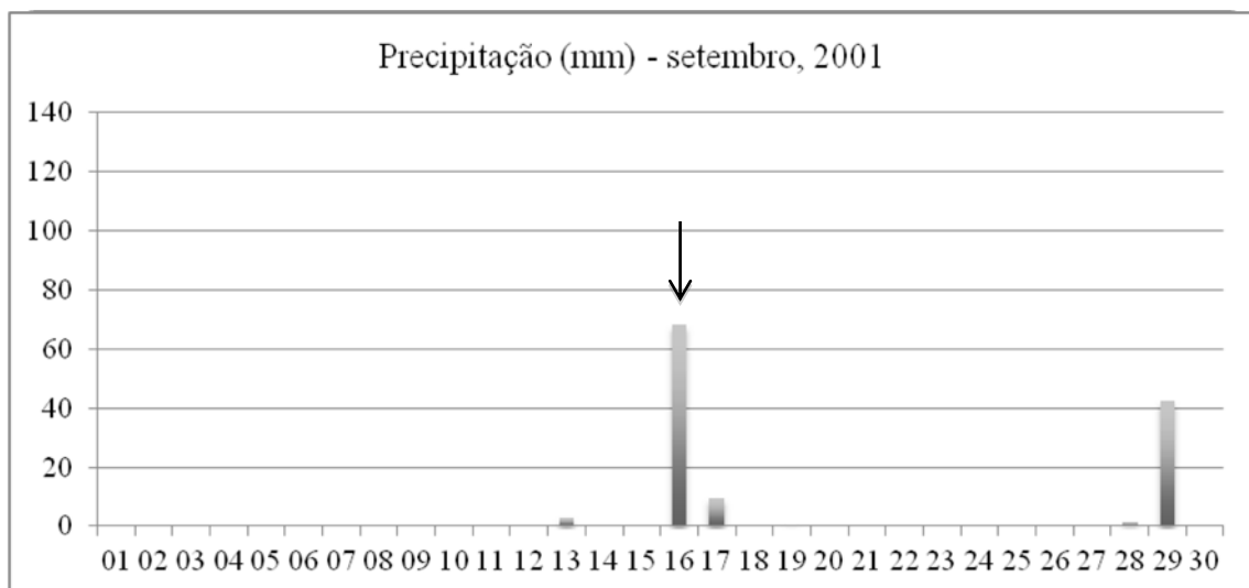
Gráfico 3 – precipitação em setembro de 2001
