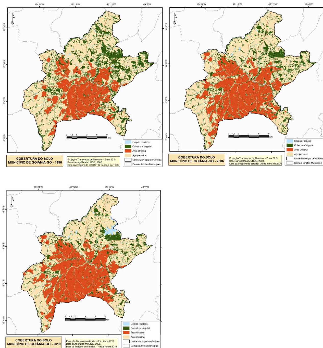
Figuras 05, 06 e 07 – Cobertura do solo em Goiânia em 1996, 2006 e 2010.
