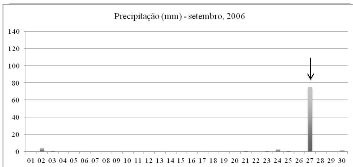
Gráfico 4 – precipitação em setembro de 2006
