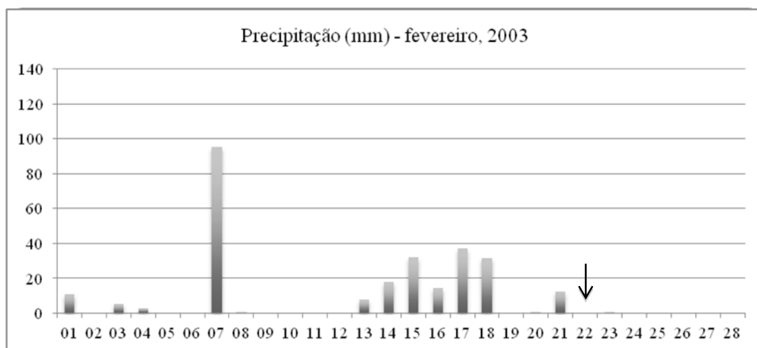
Gráfico 8 – precipitação em fevereiro de 2003
