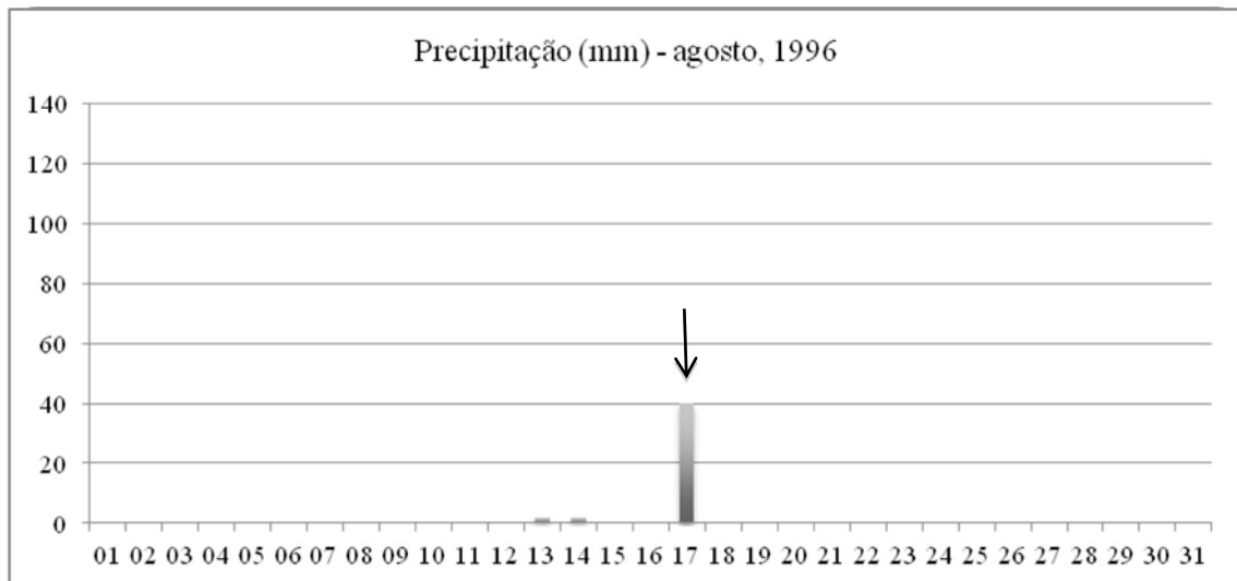
Gráfico 2 – precipitação em agosto de 1996
