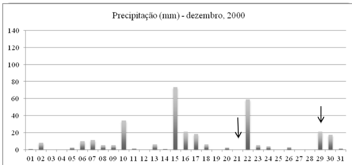
Gráfico 6 – precipitação em dezembro de 2000
