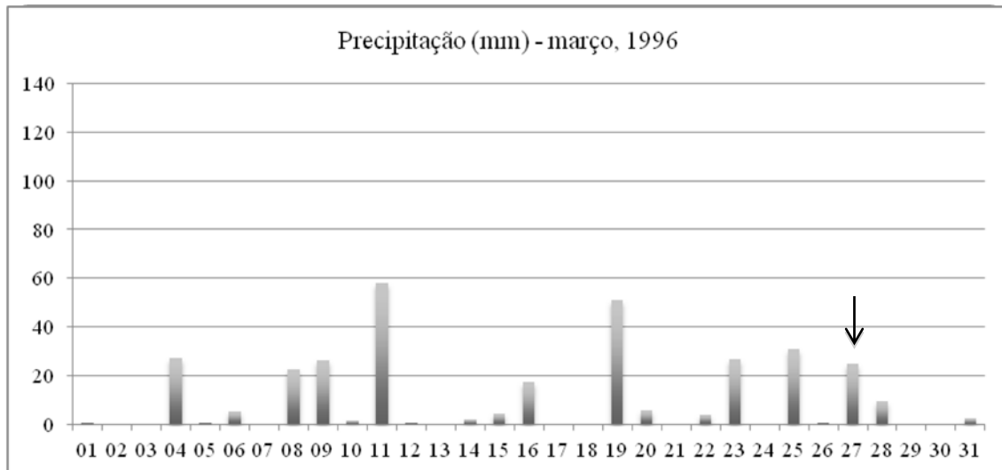
Gráfico 5 – precipitação em março de 1996
