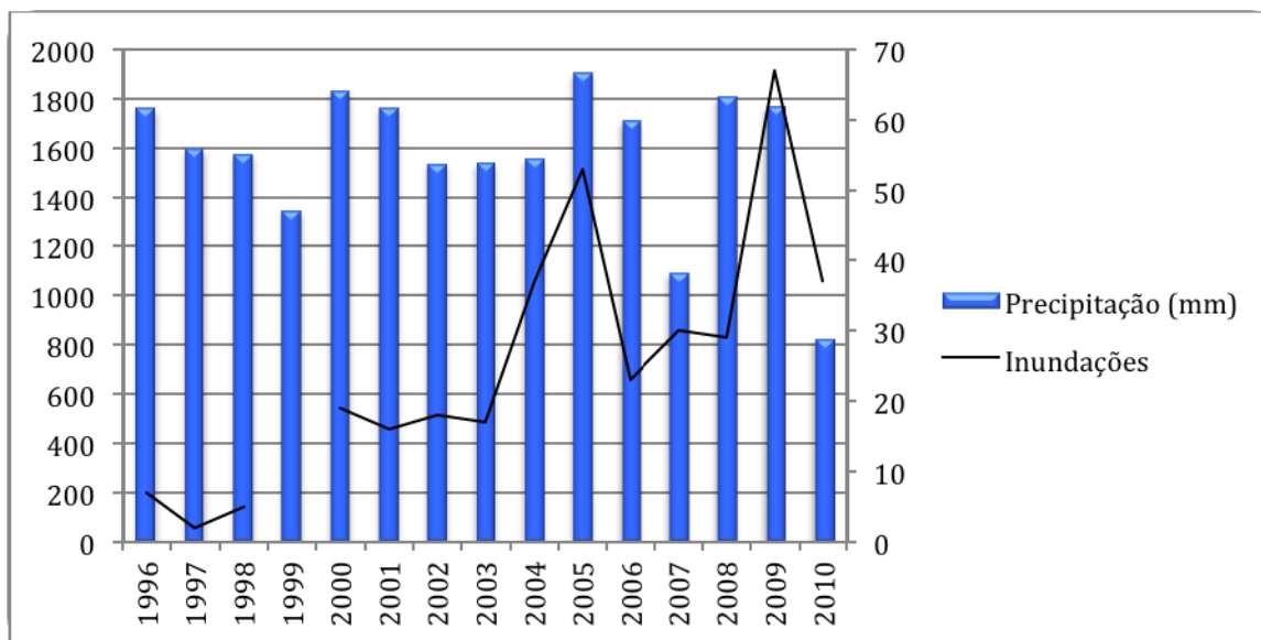
Gráfico 1 – Precipitação total anual X inundações e alagamentos, 1996 a 2010.
