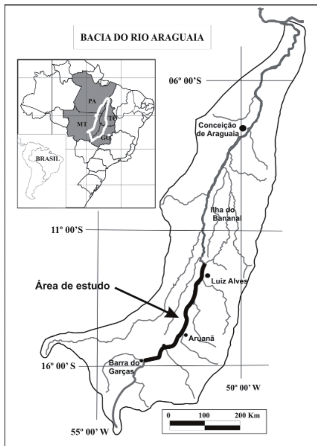
Figura 1 - Localização da área de estudo. Trecho médio curso superior do rio Araguaia e localidades.
