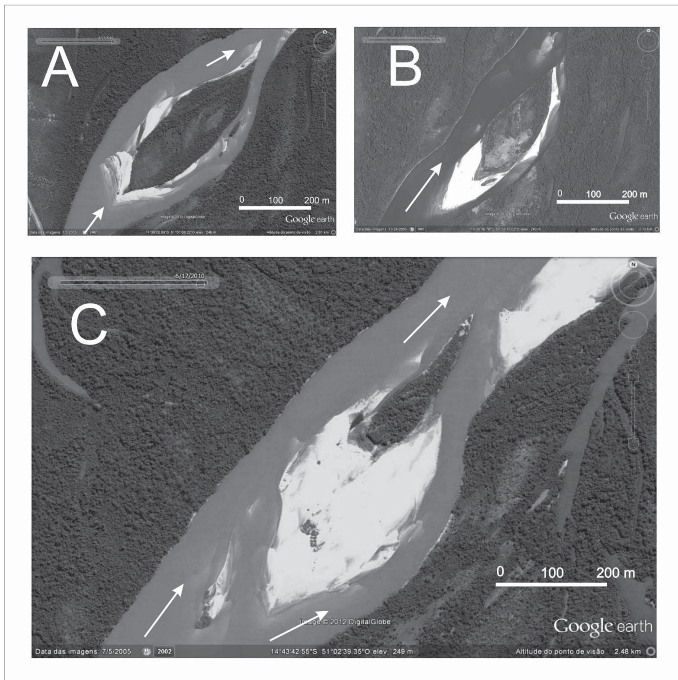
Figura 8 - Ilhas fluviais em processo de crescimento. Trechos em (A) S 14°39'20.16"/W 51°00'56.16"; (B) S 14°20'45.6"/W 50°58'20.64"; e, (C) S 14°43'39.36"/W 51°02'39.84".
