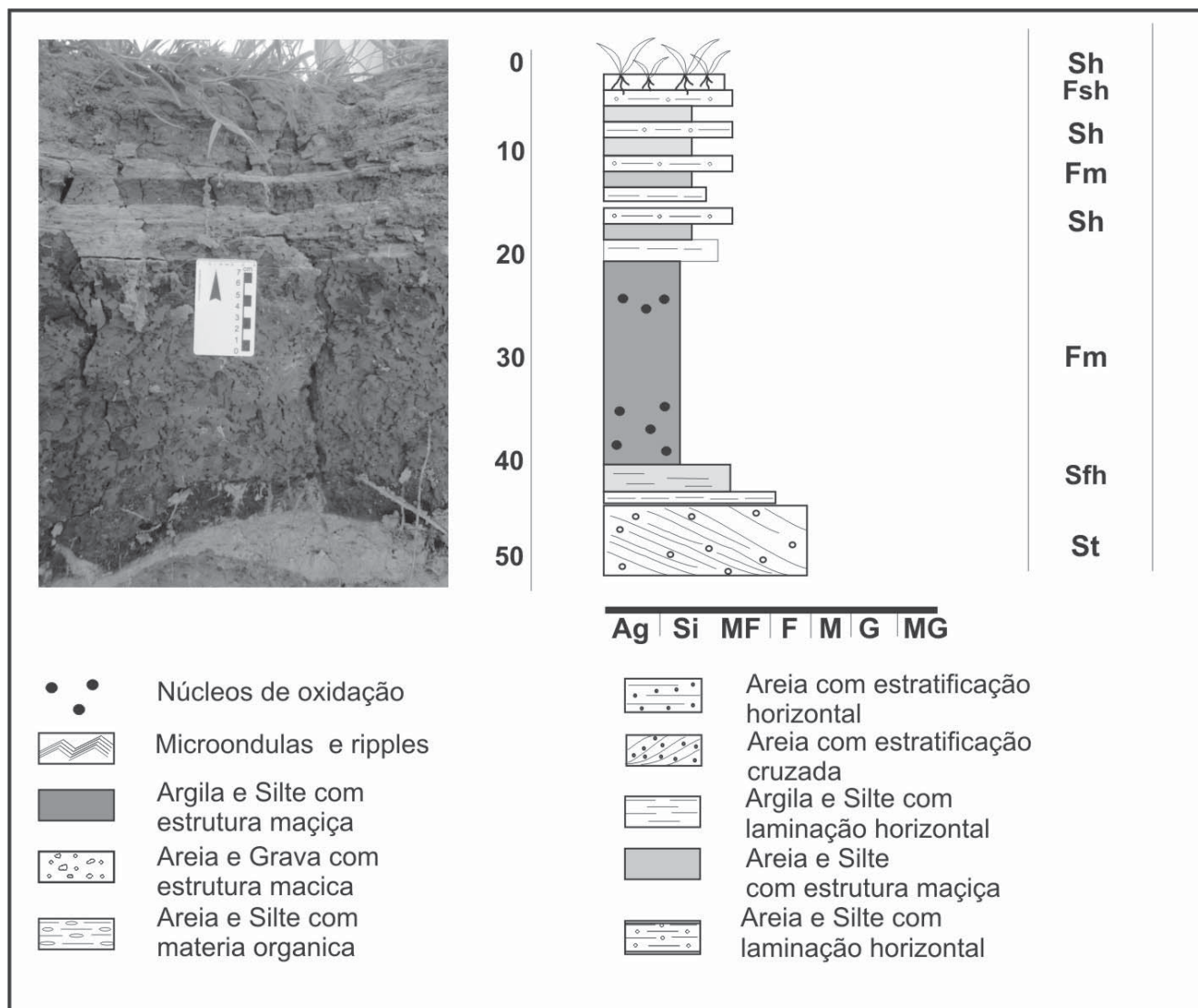
Figura 7 - Perfil da seção superior das barras laterais. Foto: Bayer/2010.
