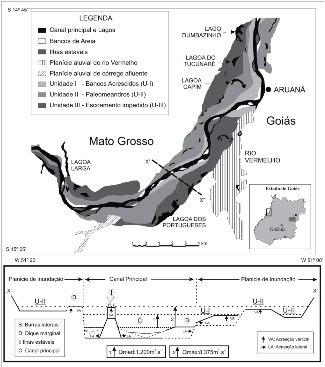
Figura 2 - Unidades geomorfológicas e croqui topográfico da planície de inundação do rio Araguaia.
