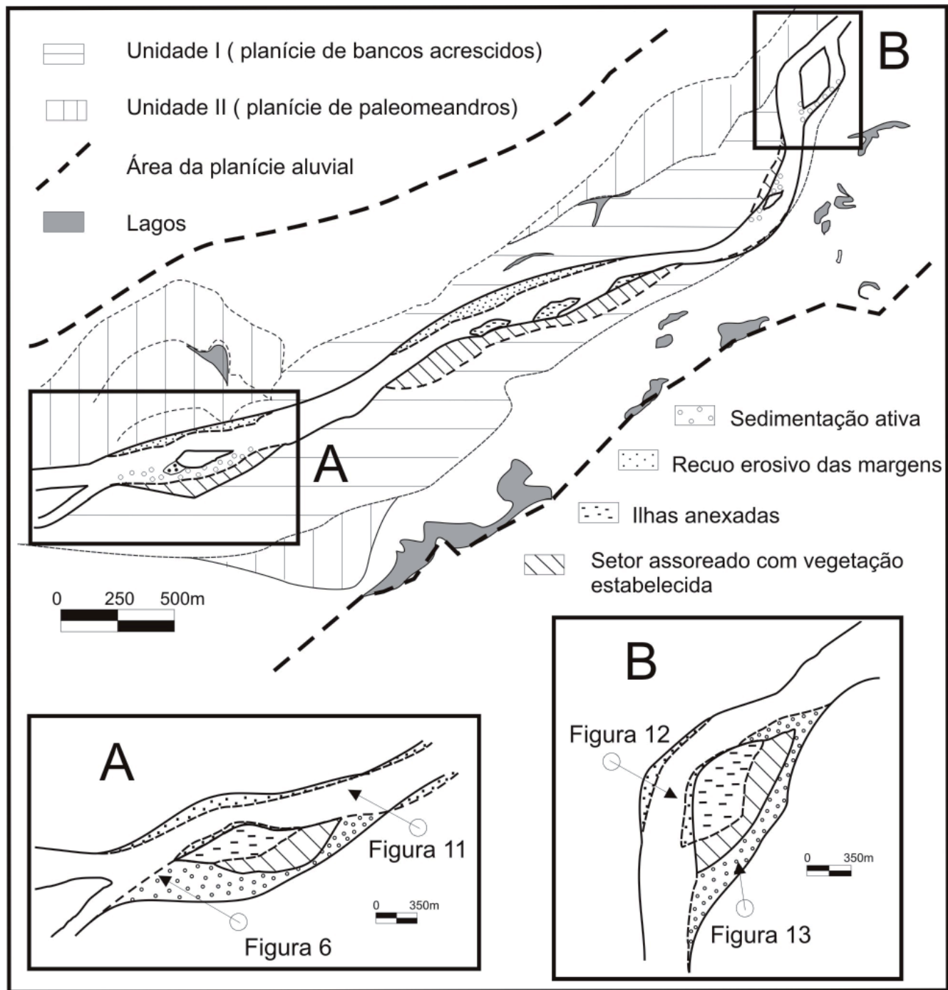
Figura 10 - Evolução morfológica de trecho do médio Araguaia.
