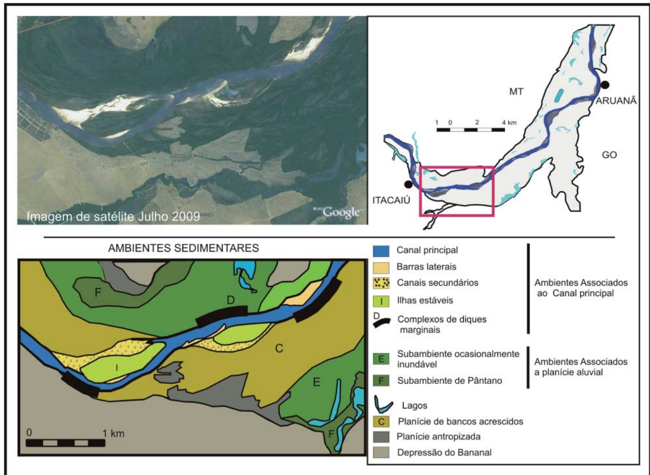
Figura 3 - Distribuição dos ambientes sedimentares na planície de inundação do rio Araguaia.
