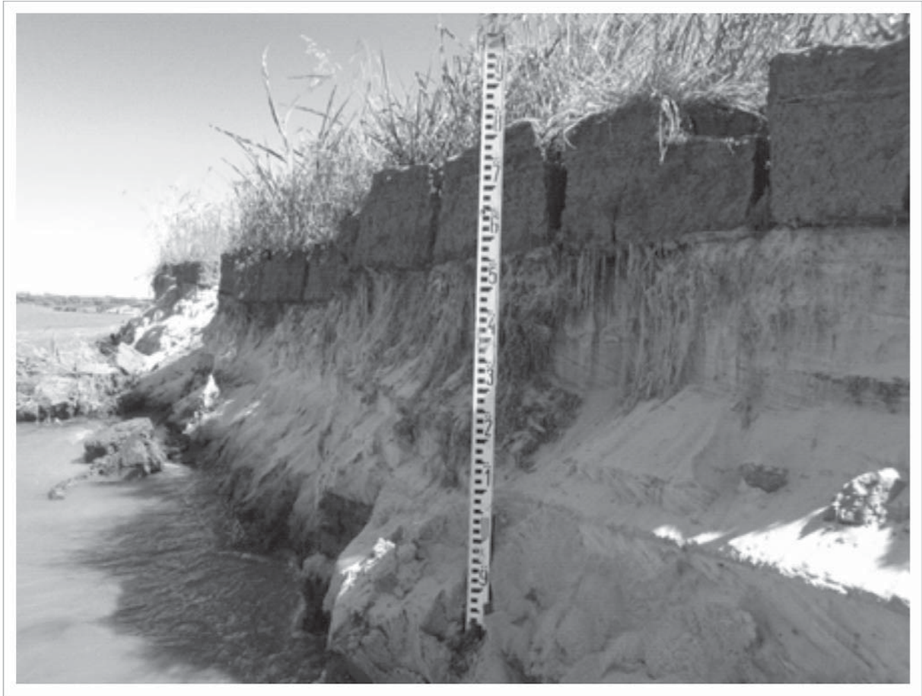
Figura 6 - Margem erosiva desenvolvida nos depósitos de uma barra lateral. Foto: Bayer/2012.
