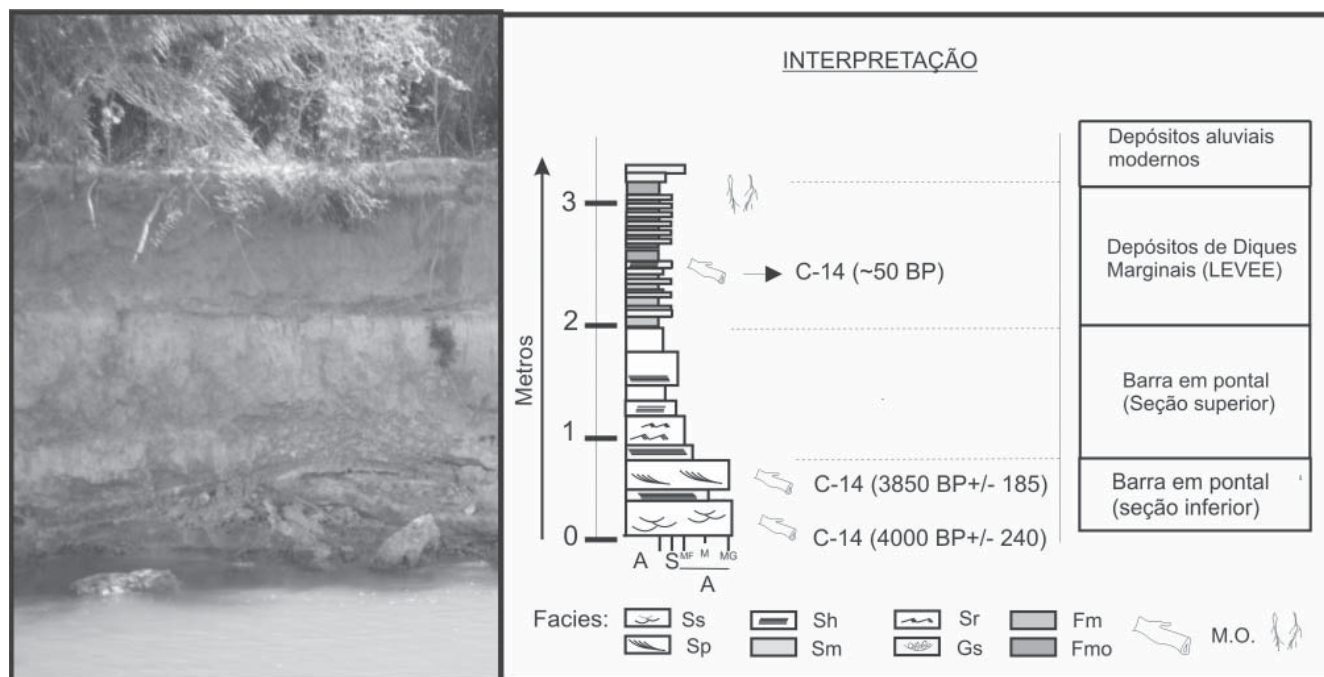
Figura 9 - Descrição do perfil do dique marginal atual (levee), sobreposto aos depósitos de canal da U-II (Paleomeandros) na margem direita do canal principal do rio Araguaia. Coord: S 14°57'54.72/ W 51°09'8.64. Foto: Bayer/2012.
