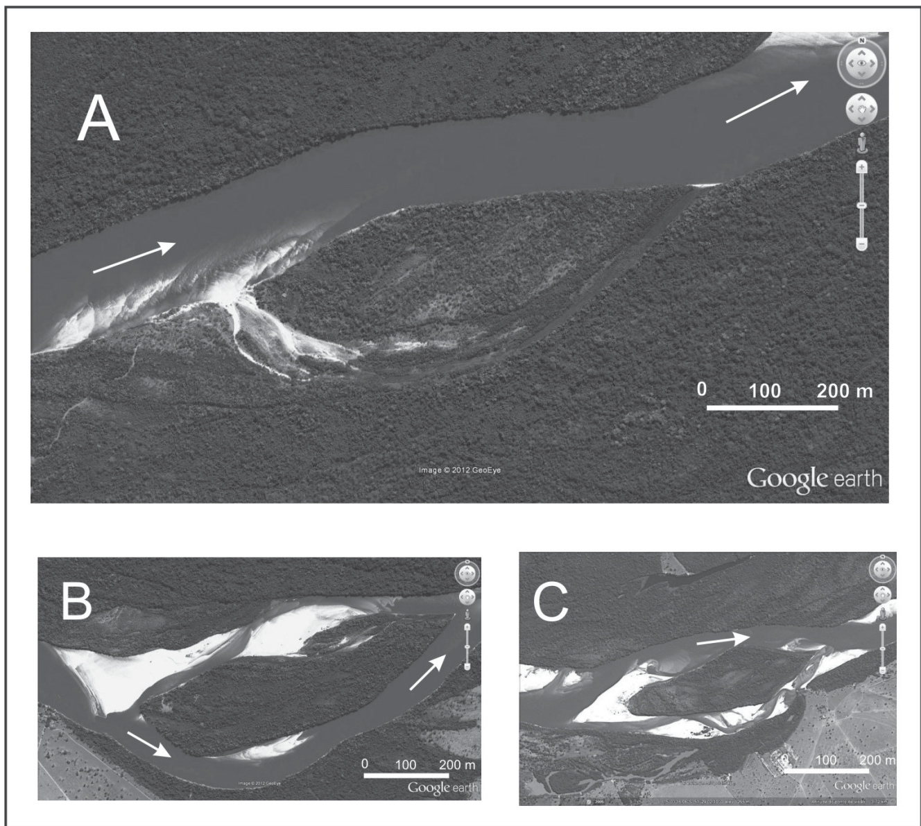
Figura 4 - Canais secundários em fases de assoreamento. Trechos em (A): S 15°01'48.12"/ W 51°14'19.62"; (B) S 15°02'39.8"/ W 51°16'3.36"; e, (C) S 15°03'31.1"/ W 51°29'0.96".
