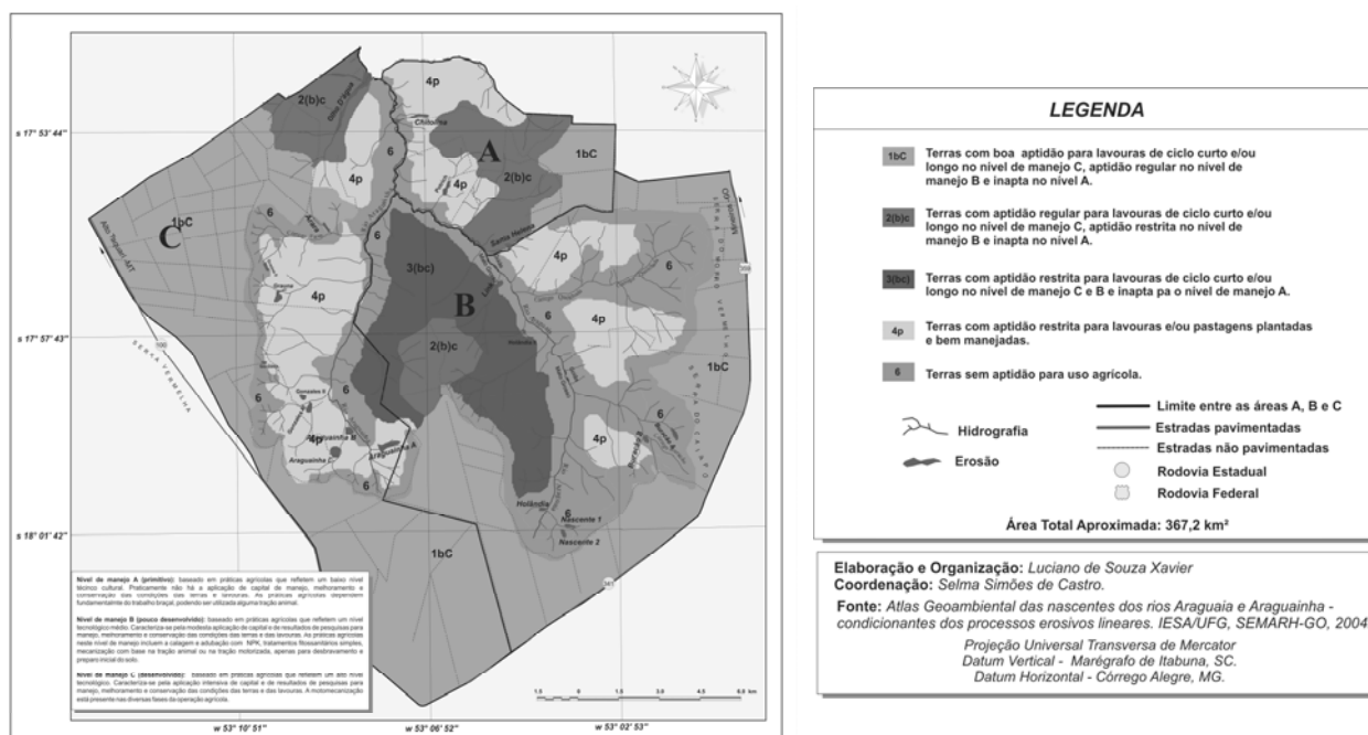
Figura 7 Aptidão agrícola das terras. Adaptado de CASTRO, XAVIER e BARBALHO (2004).
