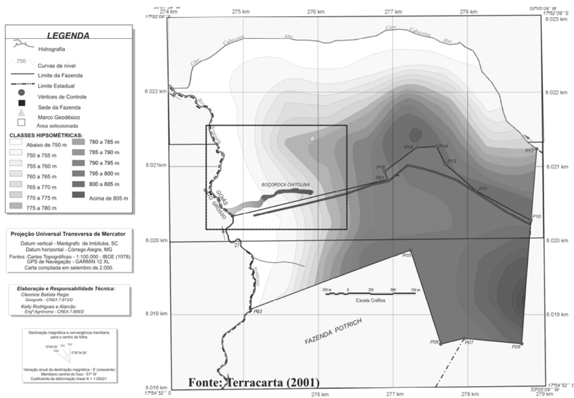
Figura 6 Vertente da Chitolina. Adaptado de TERRACARTA (2001).
