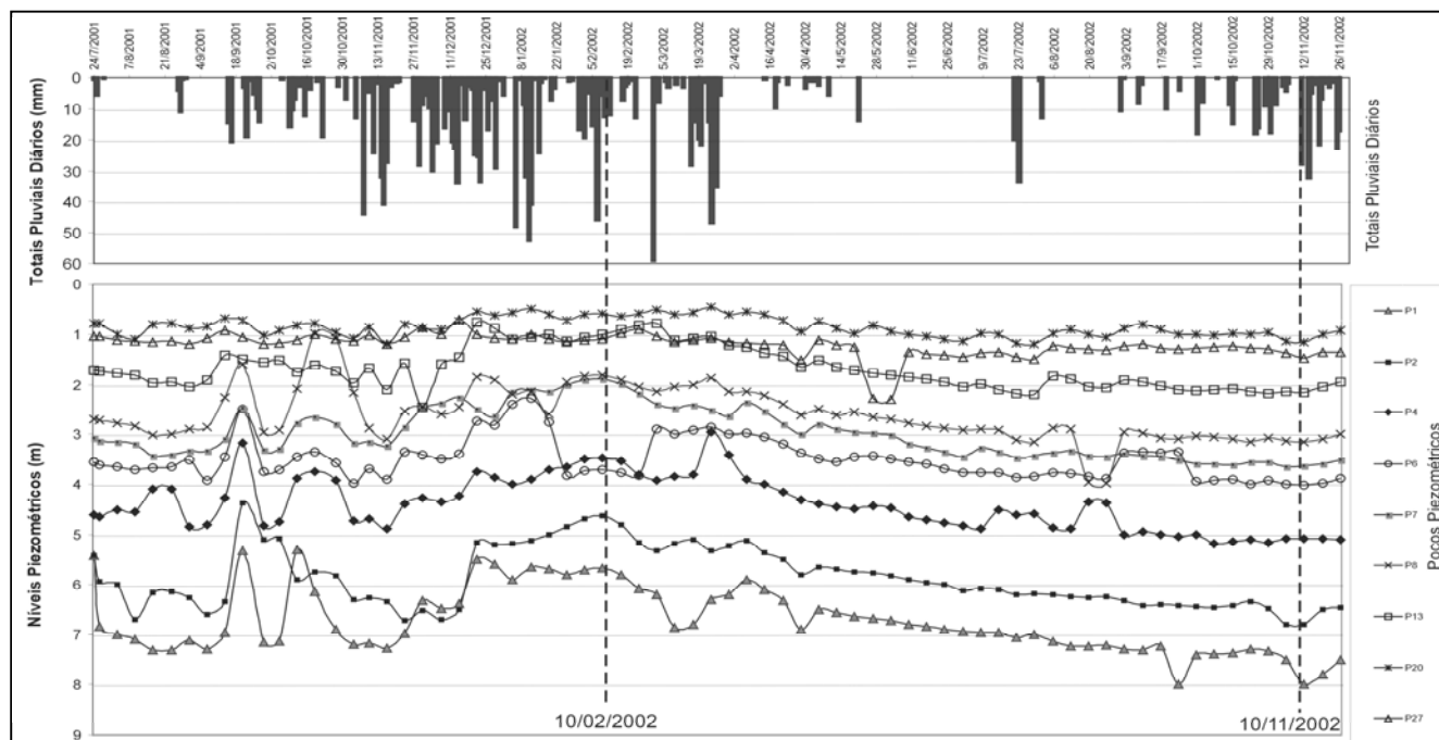
Figura 10 Pluviometria (A) e Piezometria (B) de poços representativos de montante (P1, P2), intermediários (P4, P6, P7 e P8) e de jusante (P13, 20 e P27). Adaptado de MARINHO e CASTRO (2003).
