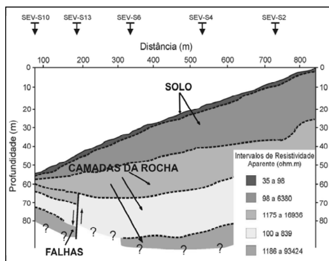
Figura 14 Seção geoeletrica agrupada, elaborada com os dados de Sondagem Elétrica Vertical, na linha da topossequência. Fonte: SHIRAIWA e MOURA (2002).
