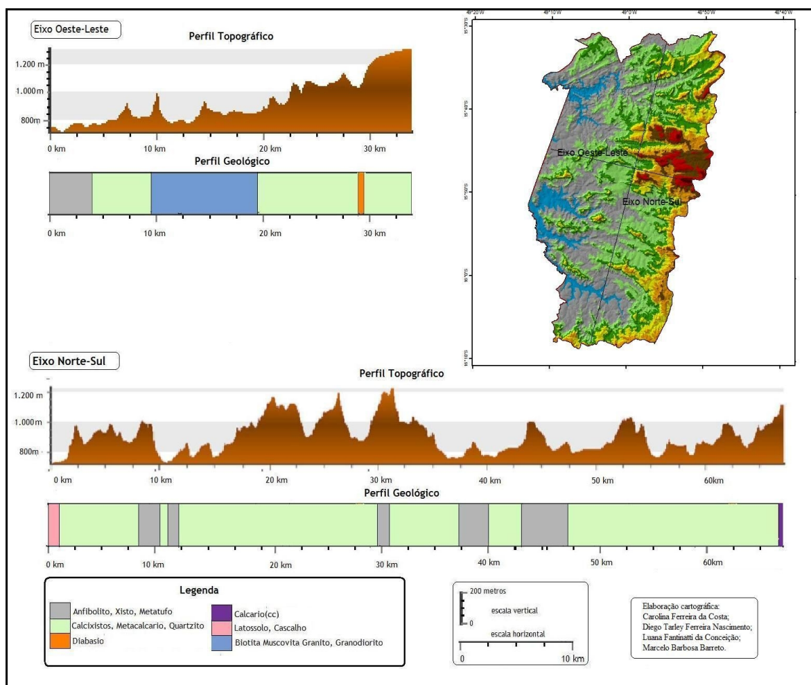
Figura 3 – Perfil topográfico e geológico de Pirenópolis
