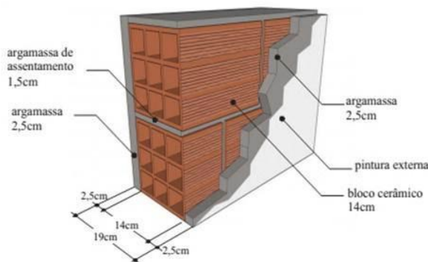
FIGURA 4: Descrição e propriedades de modelo de parede adequado para a ZB6 com bloco 14,0x19,0x29,0cm. FONTE: INMETRO (2012).
