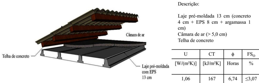
FIGURA 7: Descrição e propriedades do modelo de cobertura utilizado em Catalão e adequado para a ZB6.
