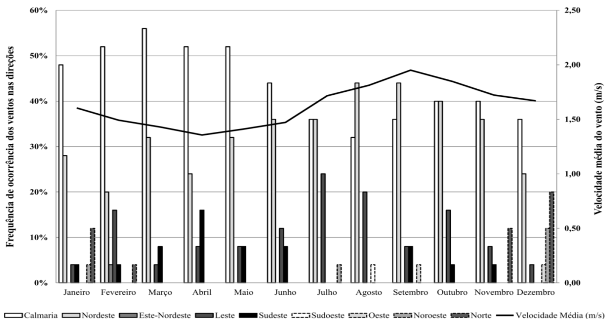
FIGURA 9: Direção predominante e velocidade média dos ventos de janeiro a dezembro de 1991 a 2015.
