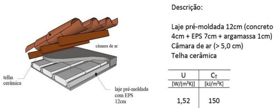
FIGURA 6: Descrição e propriedades do modelo 1 de cobertura adequado para a ZB6.
