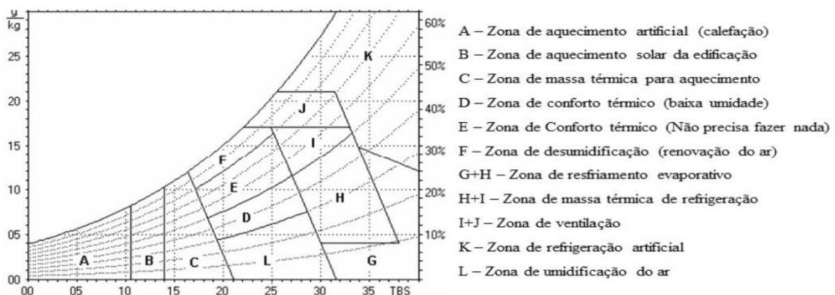
FIGURA 3: Carta bioclimática adaptada.
