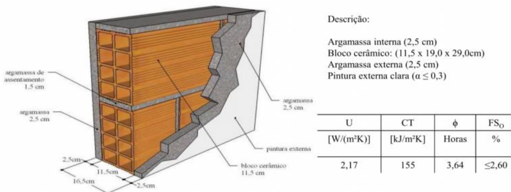
FIGURA 5: Descrição e propriedades de modelo de parede adequado para a ZB6 com bloco 11,5x19,0x29,0cm.
