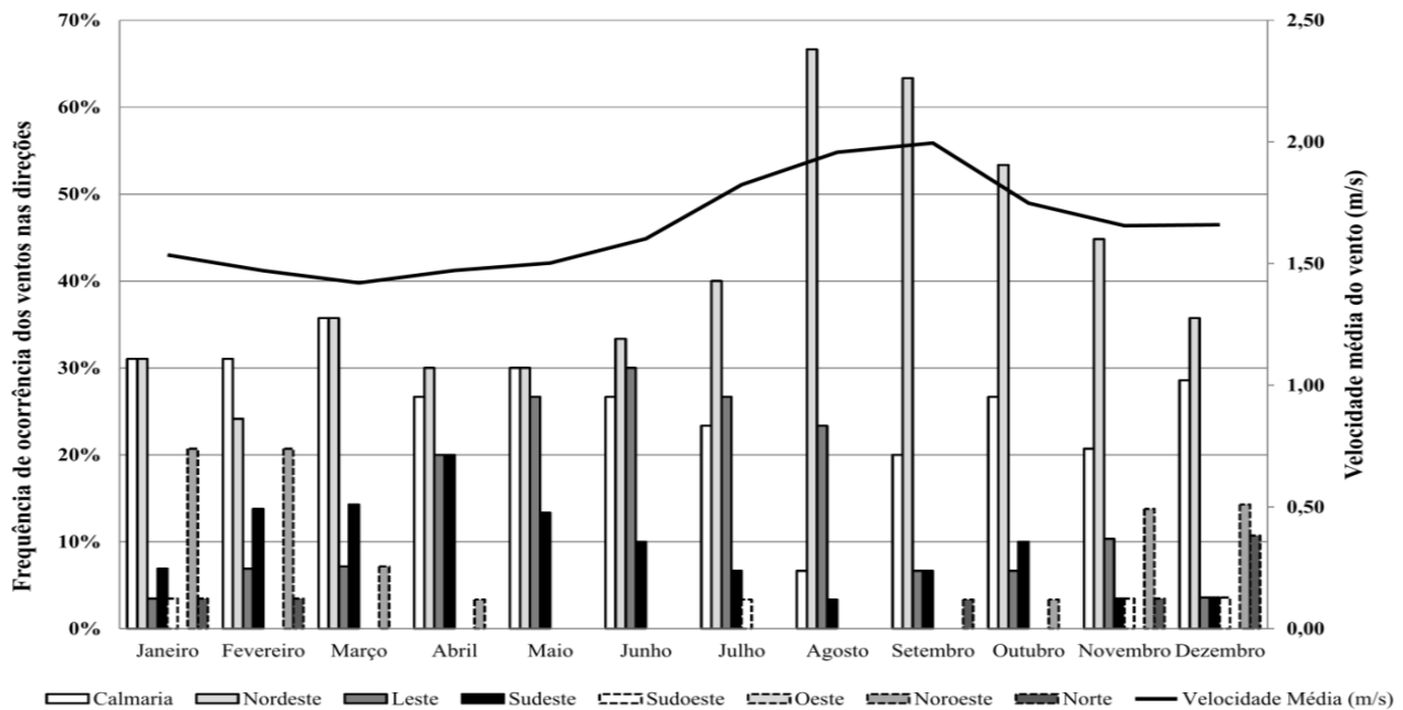
FIGURA 8: Direção predominante e velocidade média dos ventos de janeiro a dezembro de 1961 a 1990.
