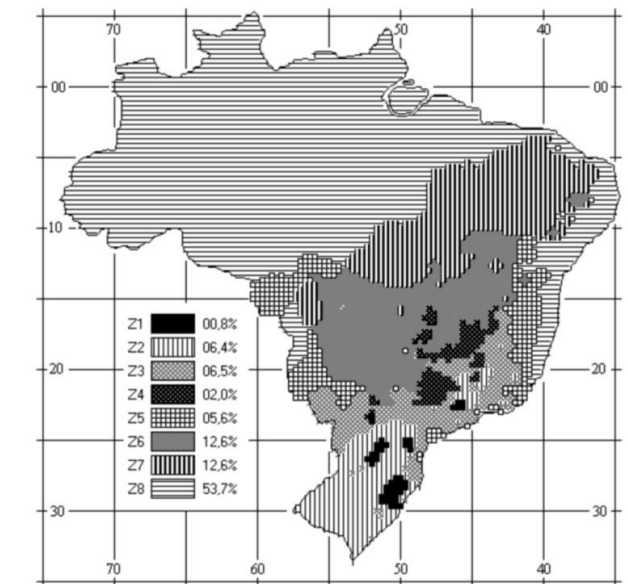
FIGURA 2: Zonas bioclimáticas brasileiras.
