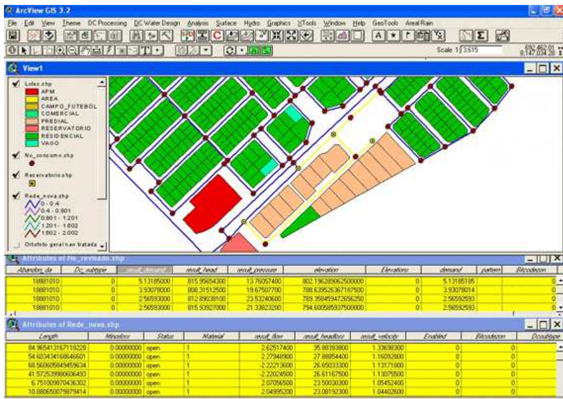
Figura 7- Área com maiores perdas de carga
