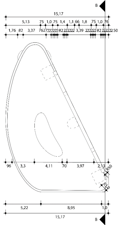
Corte A
