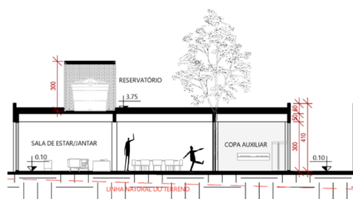
Corte DD 1 2 5 10
