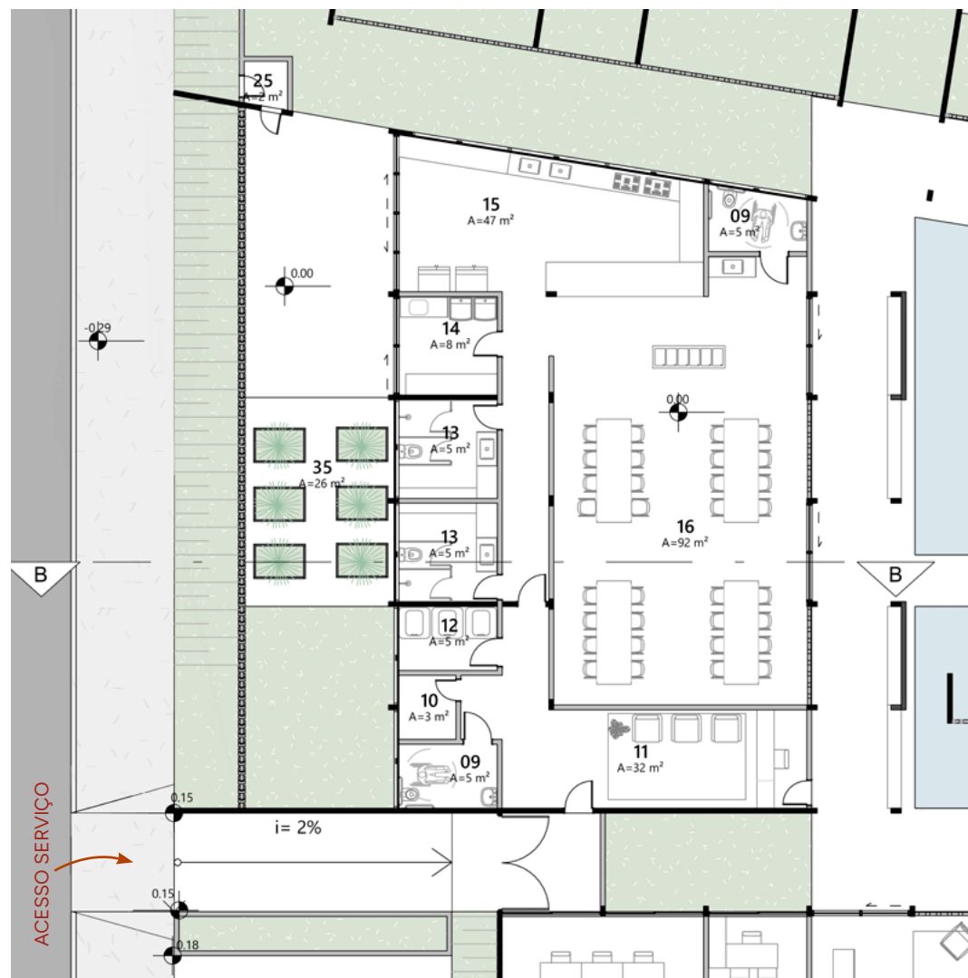
Planta baixa - Bloco serviço
