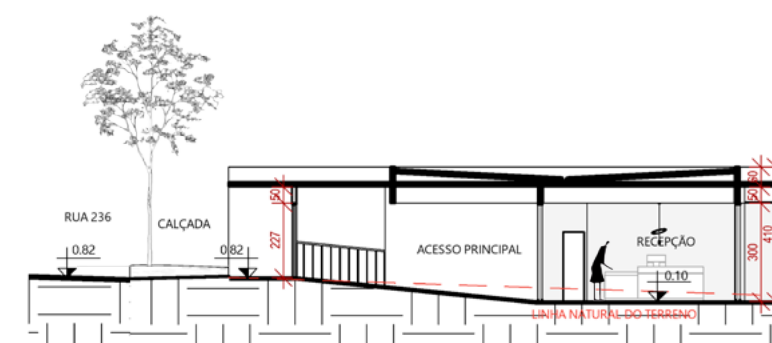
Corte EE 1 2 5 10
