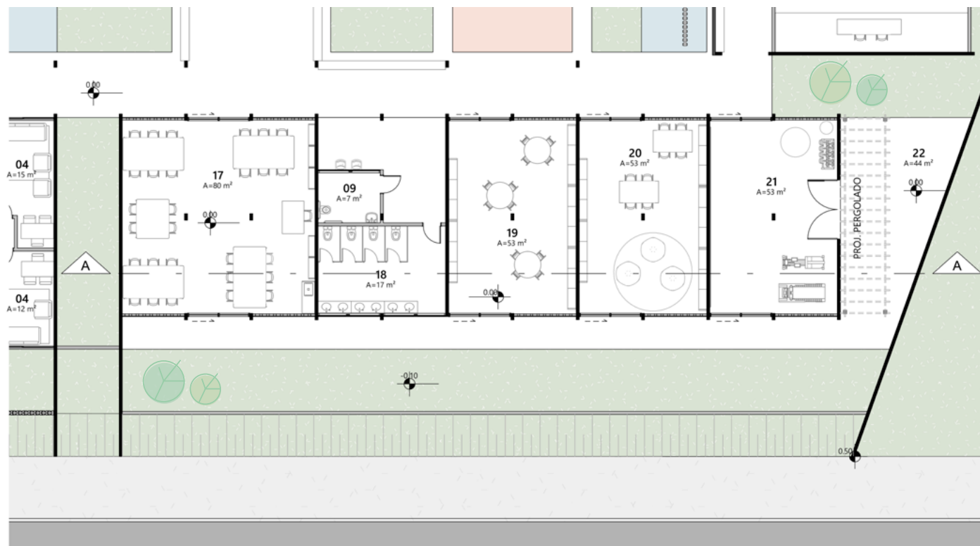
Planta baixa - Bloco ateliê
