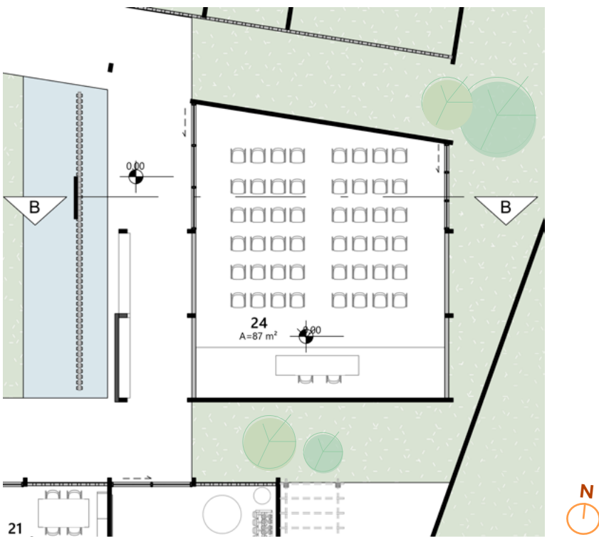
Planta baixa - Bloco auditório
