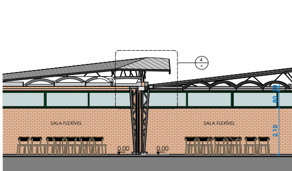
Fig . 101- Corte HH. Escala 1:200
