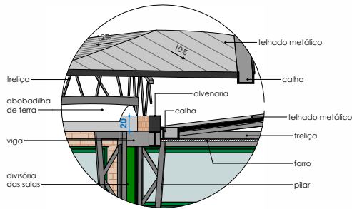
Fig . 102- Detalhe cobertura. Escala 1:50
