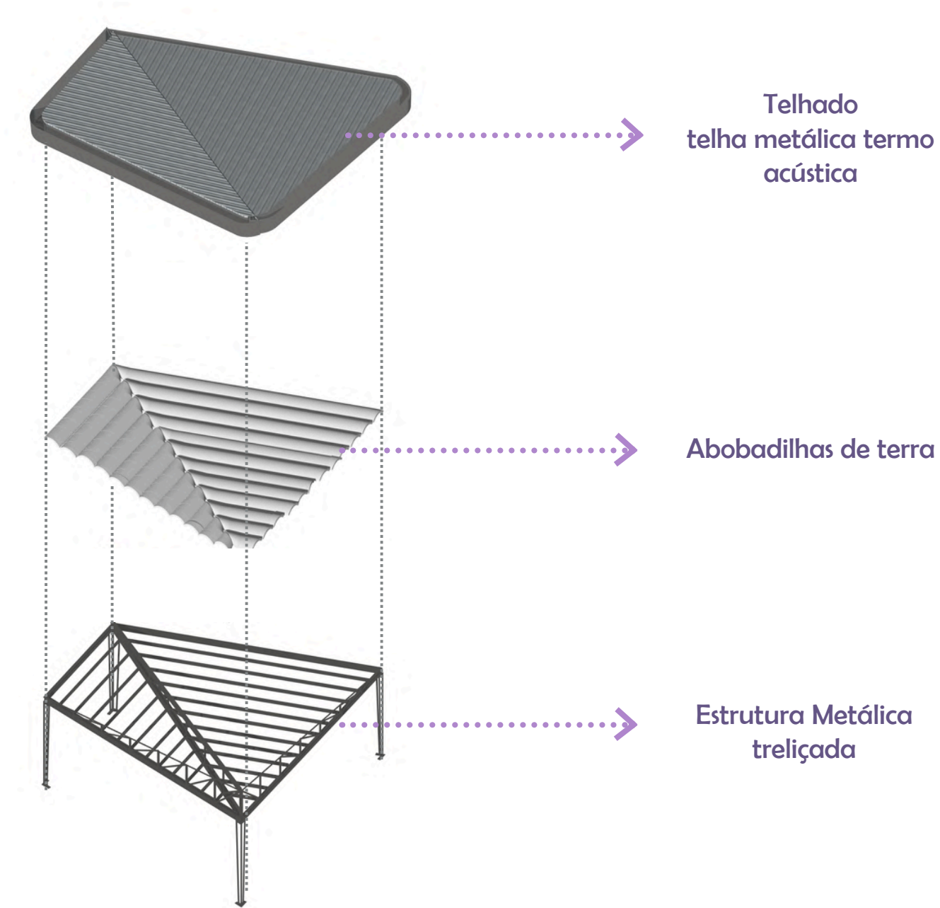
Fig . 107- Diagrama estrutura Fonte: Elaboração própria.
