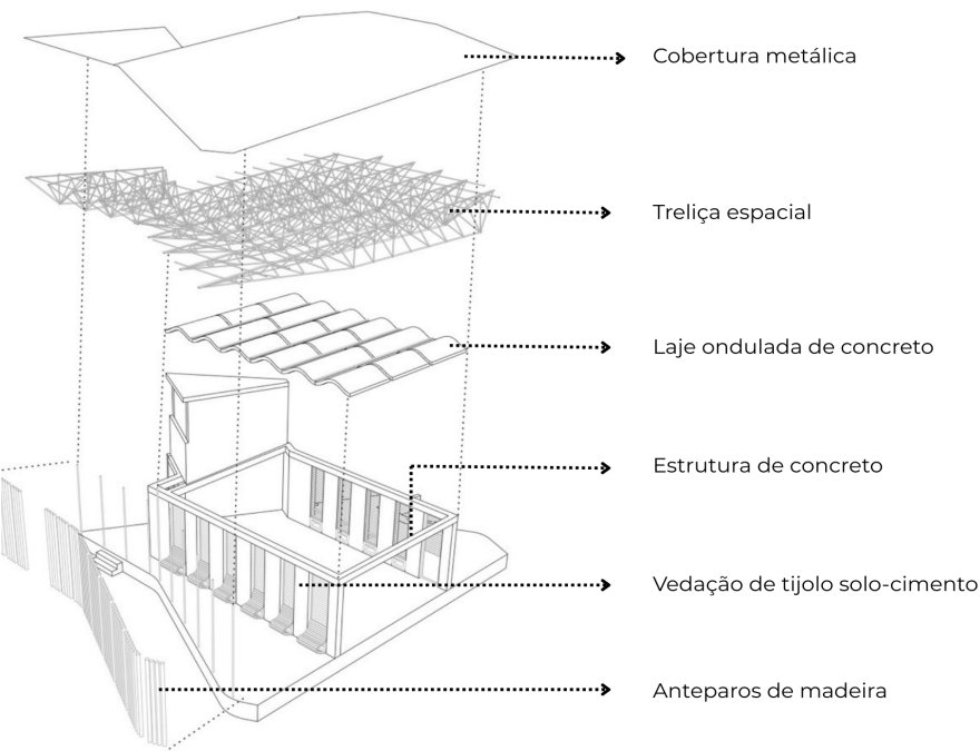
Fig. 49 e 50- Estrutura da escola. Modificado pela autora. Disponível em: https://www.archdaily.com.br/01-158650/centro-de-oportunidade-para-mulheres-slash-sharon-davis-design . Acesso em: 06 out. 2025
