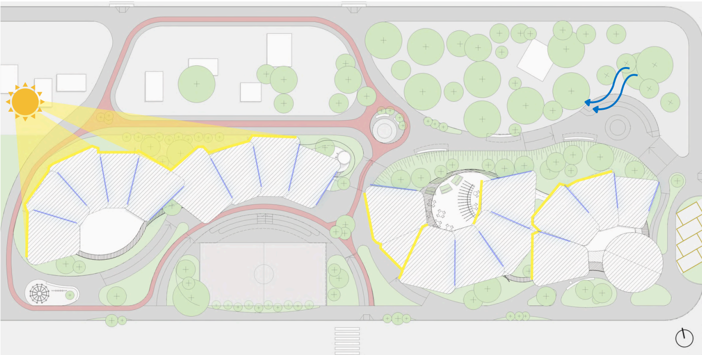
Fig . 103- Diagrama insolação. Fonte: Elaboração própria.
