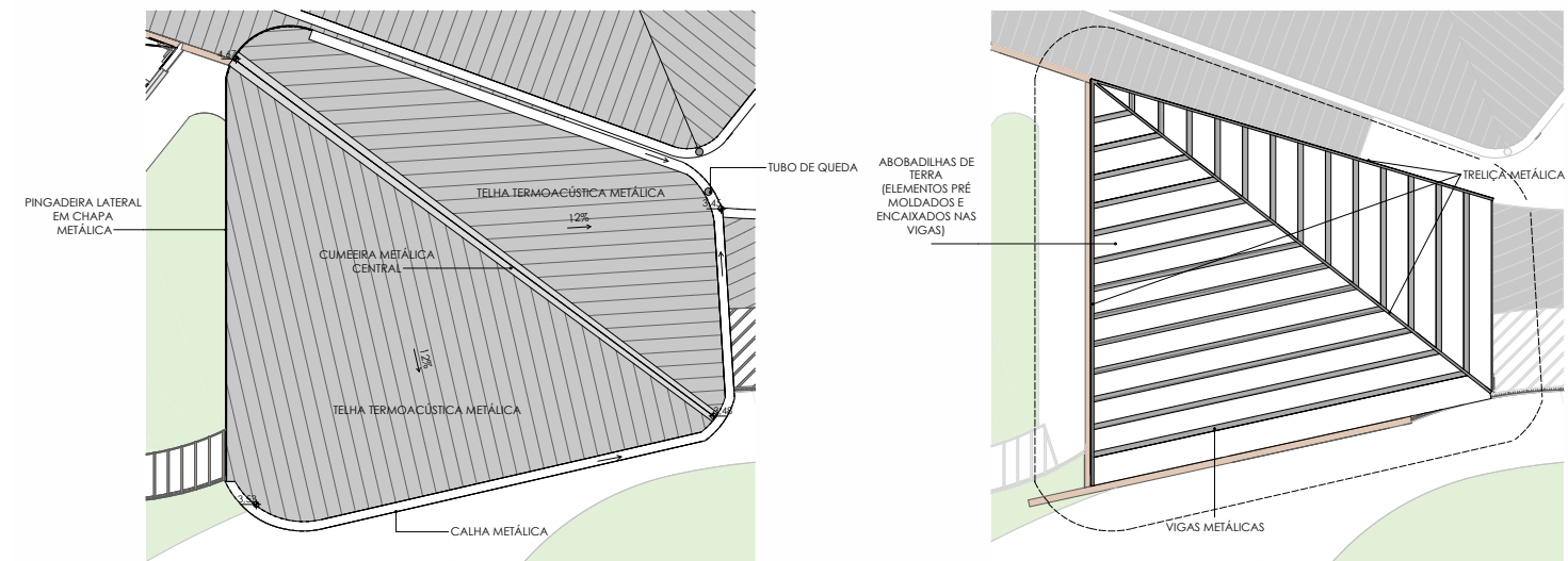
Fig . 108 e 109- Detalhes cobertura. Escala 1: 200
