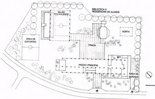
Fig. 33- Implantação do CIEP. Disponível em: O-Livro-dos-CIEPs-por-Darcy-Ribeiro.pdf. Acesso em: 06 out. 2025
