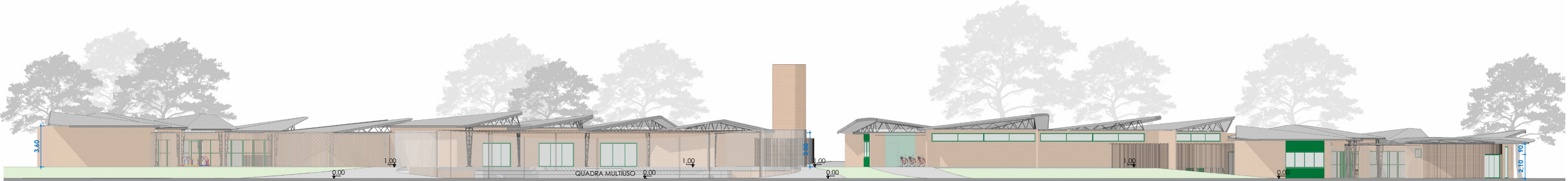
Fig . 92- Corte BB. Escala 1: 350
