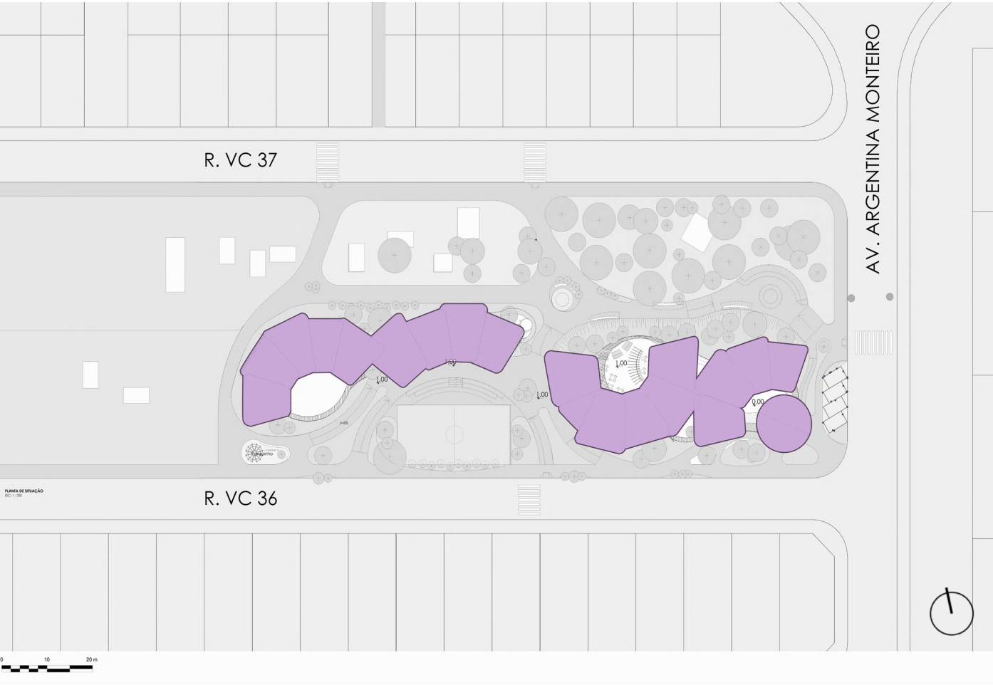
Fig . 88- Planta de situação. Escala 1: 1000
