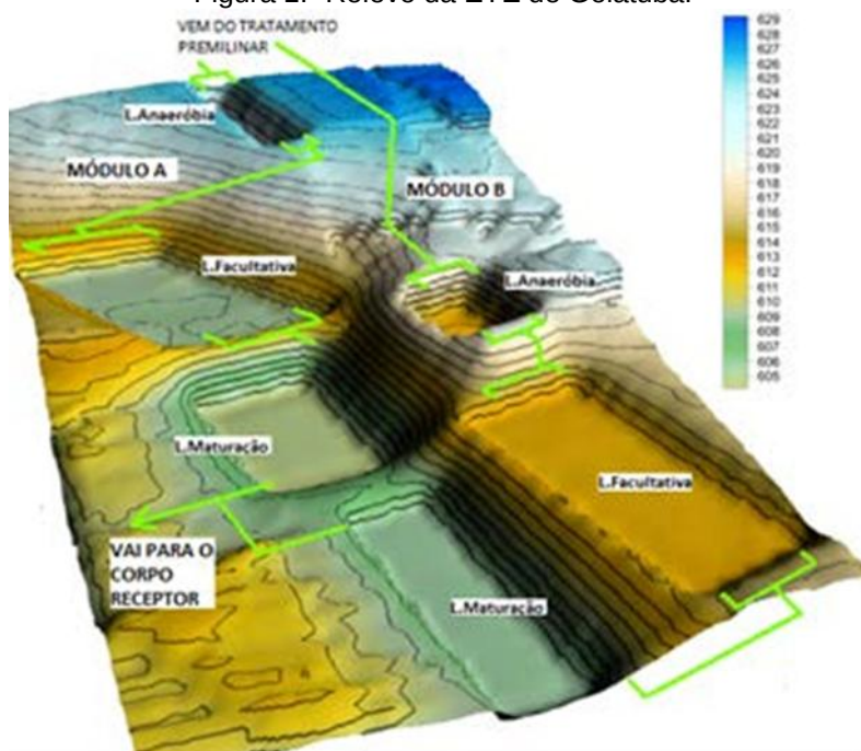
Figura 1.- Relevo da ETE de Goiatuba.
