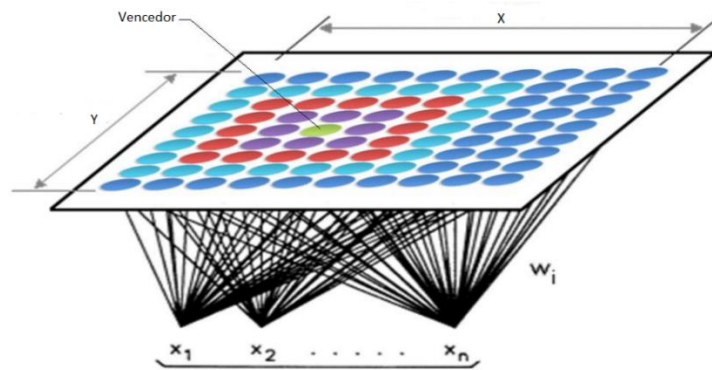
Figura 9 - Vetor de entrada x conectado ao Mapa Auto-Organizável por meio do vetor de pesos w_i
