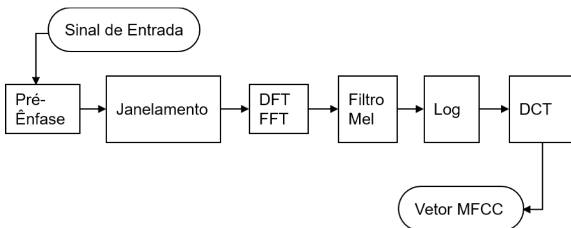
Figura 6 – Etapas do método MFCC
