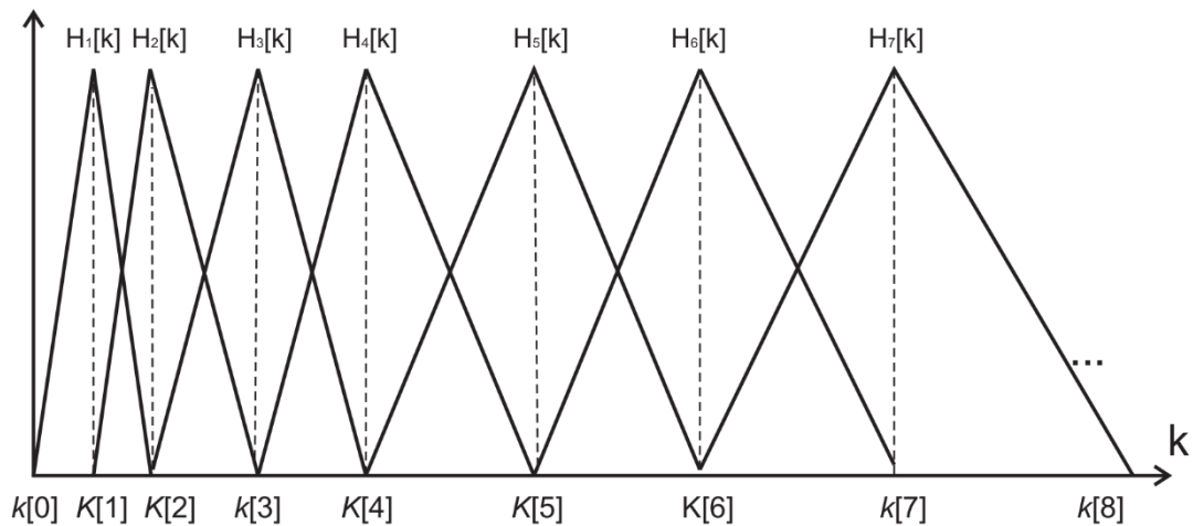
Figura 7 – Banco de filtros usado no método MFCC
