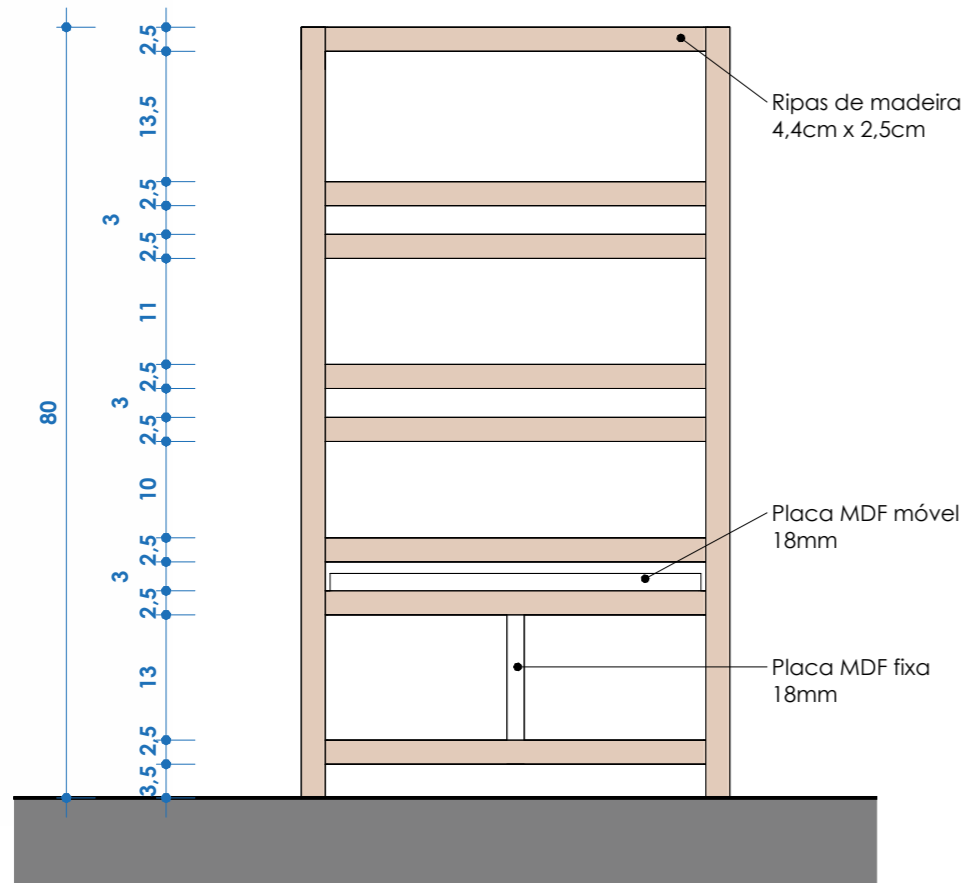
Corte 1 ESC: 1 : 10
