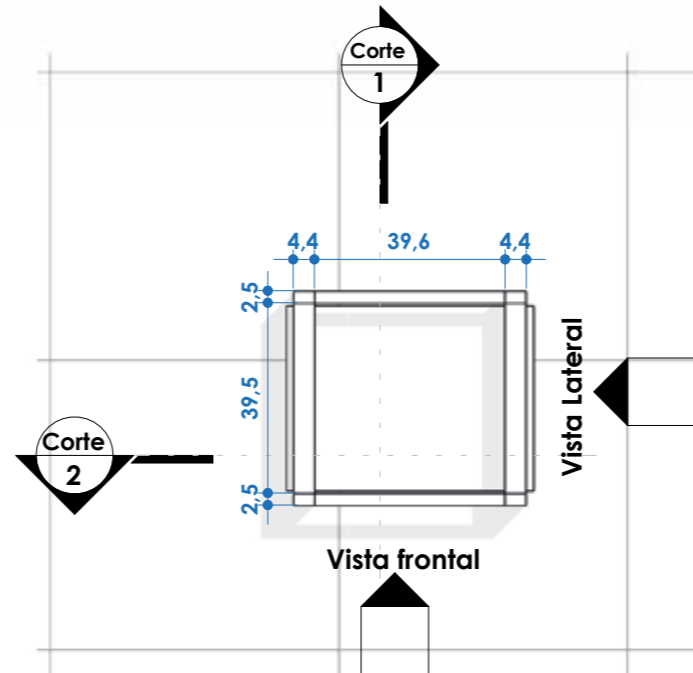
Vista superior ESC: 1 : 20
