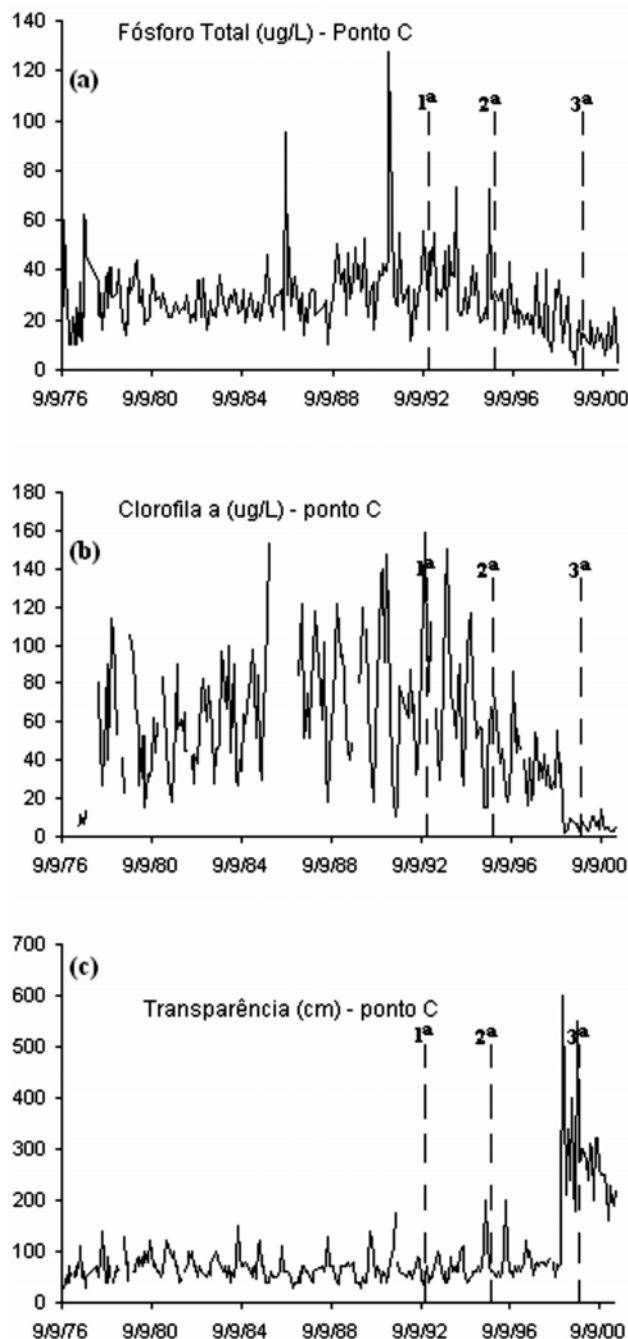
Figura 4. Variação de Fósforo Total ( \mu\text{g}\cdot\text{L}^{-1} ), Clorofila-a ( \mu\text{g}\cdot\text{L}^{-1} ) e Transparência (cm) para o corpo central (ponto C) do Lago Paranoá. 1ª intervenção: 01/1993; 2ª intervenção: 01/1996; 3ª intervenção: 11/1999.
