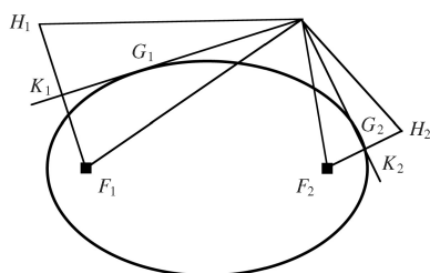
Figura 3.3: Triângulos isósceles
