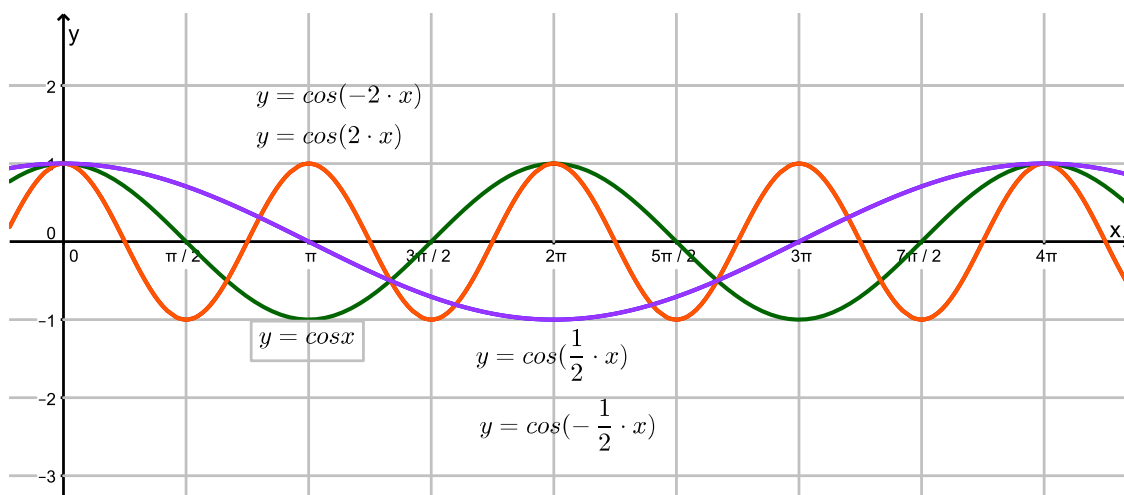
Figura 12: f(x) = \cos x Comparada com f(x) = \cos(cx)
