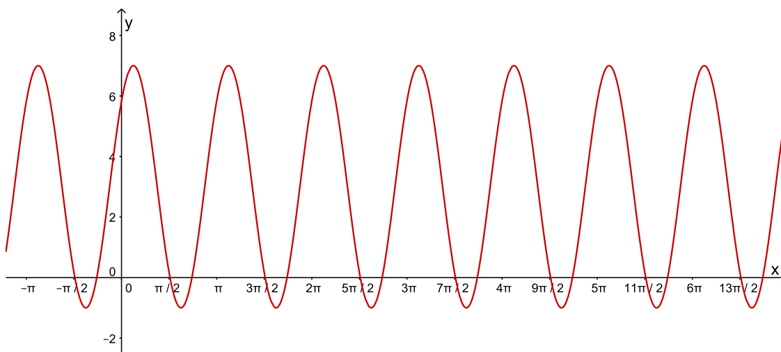
Figura 8: Gráfico de f(x) = 3 + 4\text{sen}(2x + \frac{\pi}{4})
