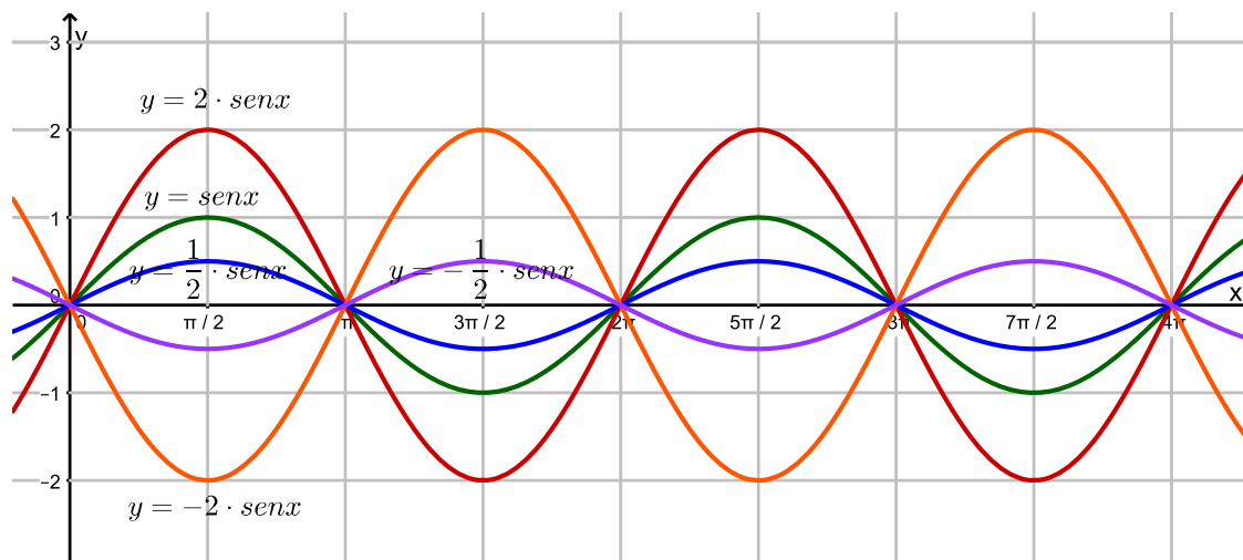
Figura 4: f(x) = \text{sen } x Comparada com f(x) = b \text{sen } x
