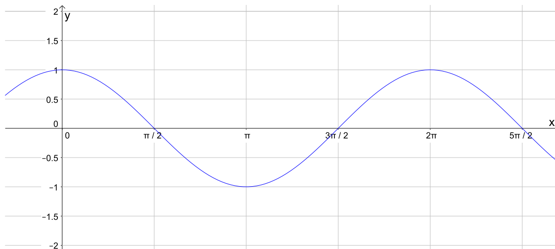
Figura 9: f(x) = \cos x
