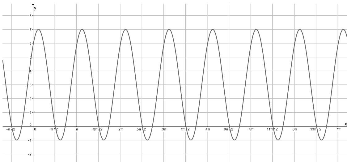
Figura 15: Gráfico de f(x) = 3 + 4 \cos(2x - \frac{\pi}{4})
