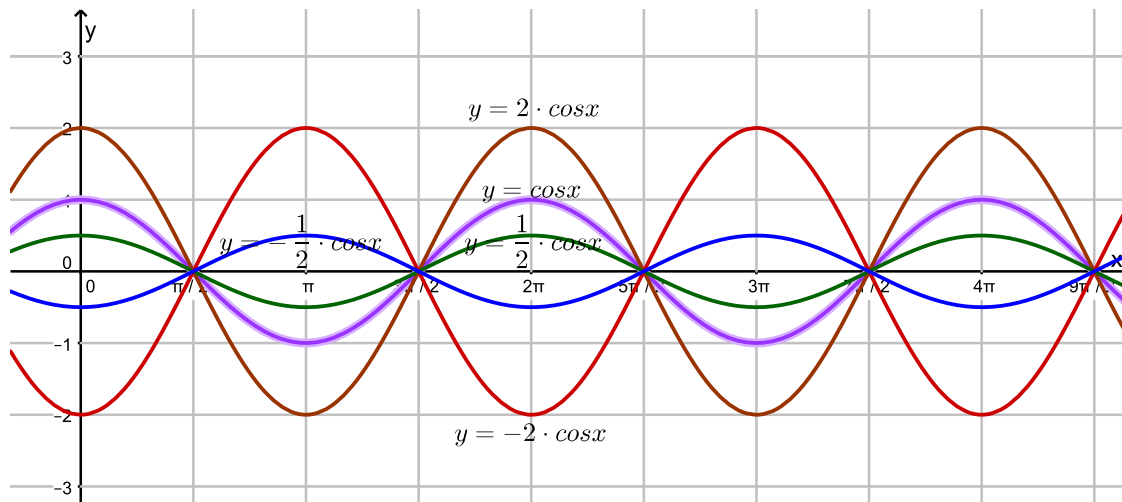
Figura 11: f(x) = \cos x Comparada com f(x) = b \cos x
