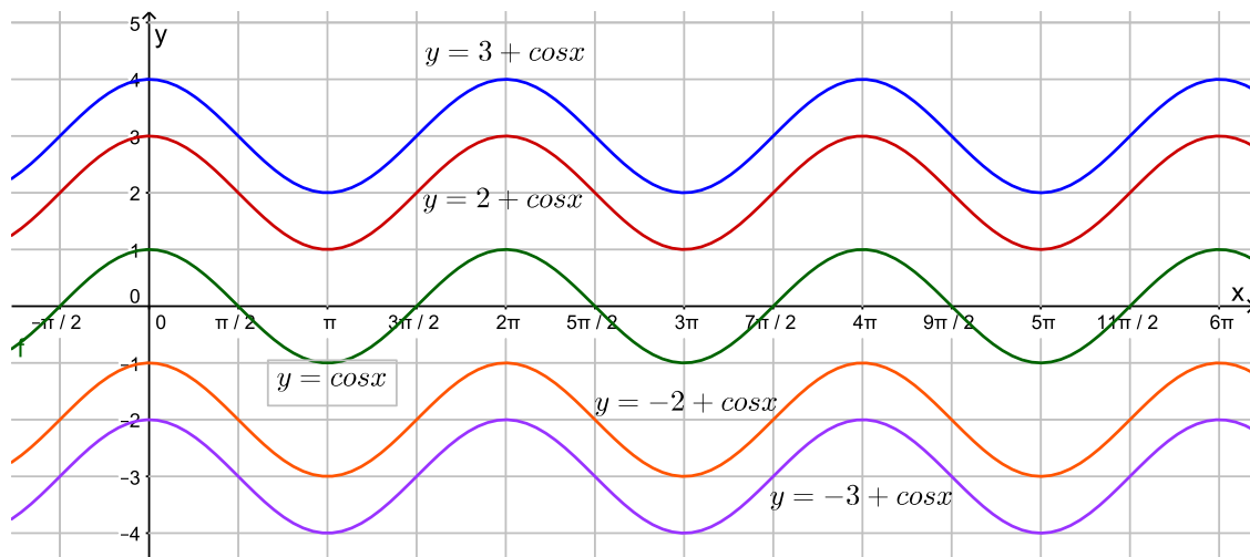
Figura 10: f(x) = \cos x Comparada com f(x) = a + \cos x
