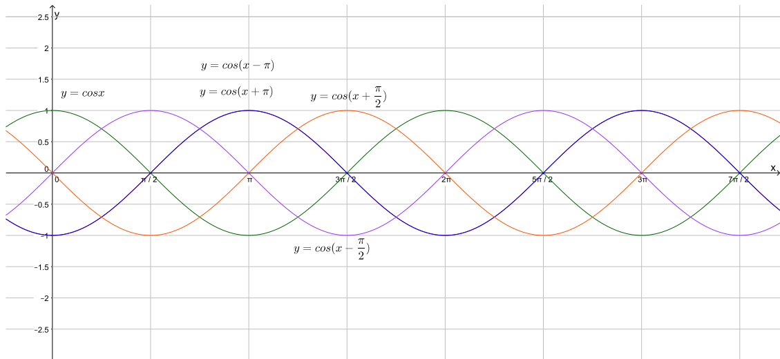
Figura 14: f(x) = \cos x Comparada com f(x) = \cos(x + d)
