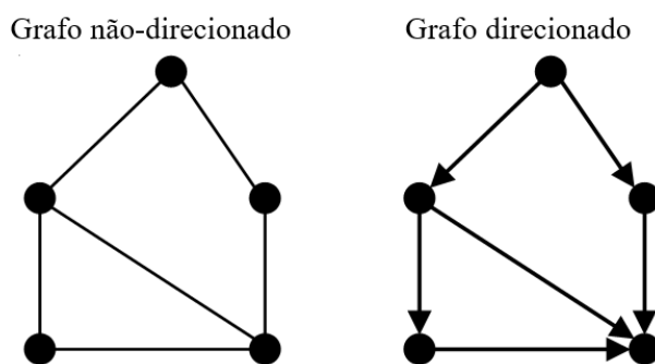
Figura 7 - Exemplos de Grafos simples
