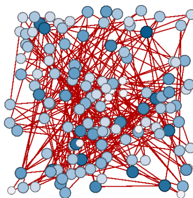
Figura 8 – Exemplo de Grafo complexo
