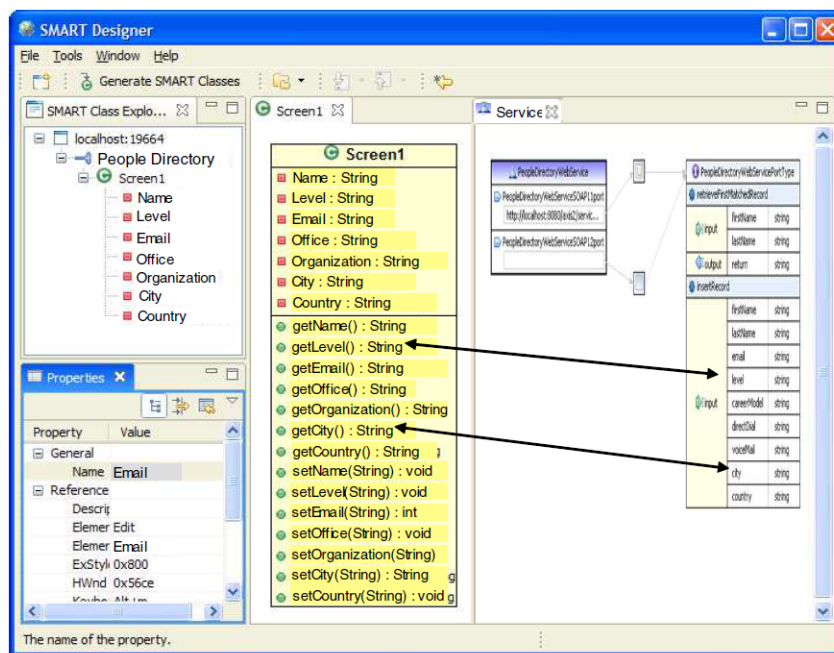
Figura 6.3: Visualização de Conroy et al. (2007) (reusado com permissão de Conroy et al. (CONROY et al., 2007))
