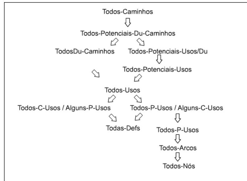
Figura 2.1: Ordem parcial entre os critérios Potenciais-Usos básicos, Critérios de fluxo de dados e de fluxo de controle (MALDONADO, 1991).
