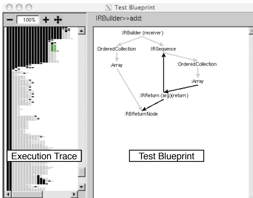
Figura 6.4: Visualização de (LIENHARD et al., 2008) mostrando o trace de execução e a parte o blueprint do teste (reusado com permissão de Lienhard et al. (2008))
