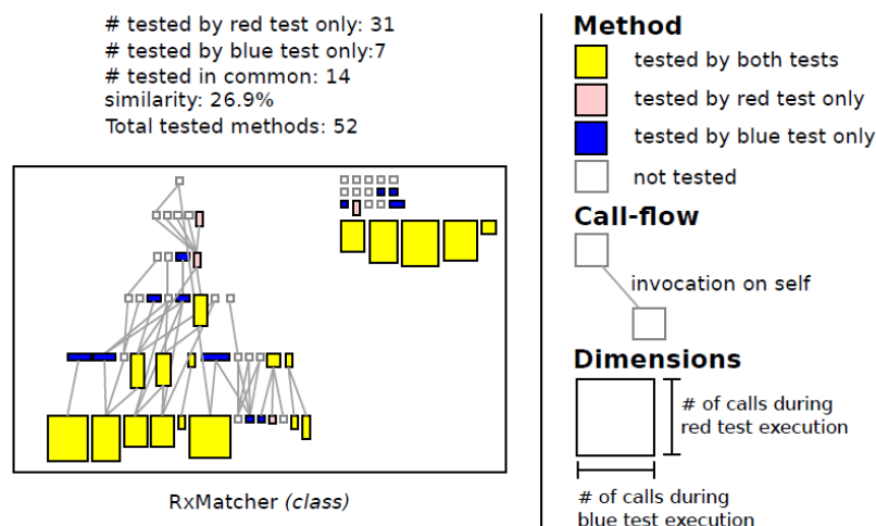
Figura 6.2: Blueprint de Estefo (2012) mostrando as diferenças entre um par de execuções de casos de teste (reusado com permissão de Estefo (2012) )
