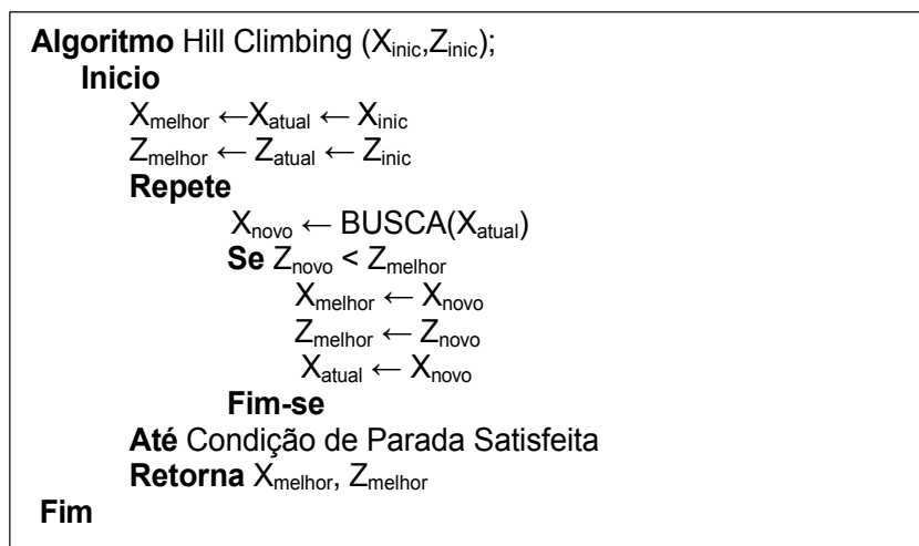
Figura 3.3 – Algoritmo HC
