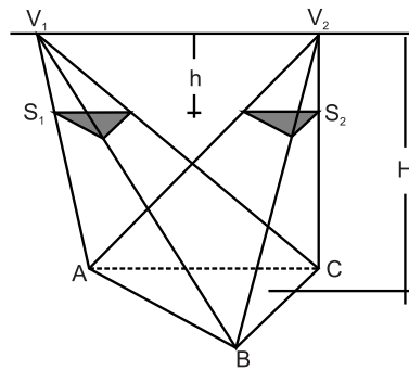
Figura 11: Volumes iguais
