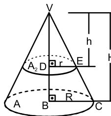
Figura 19: Razões entre as áreas
