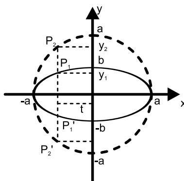
Figura 31: Elipse e Circunferência
