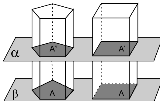
Figura 5: Áreas equivalentes
