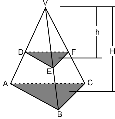
Figura 9: Triângulos Semelhantes
