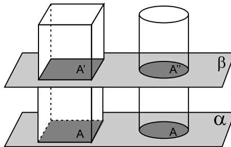
Figura 7: Aplicando o Princípio de Cavalieri
