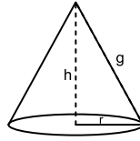
Figura 17: Elementos de um cone
