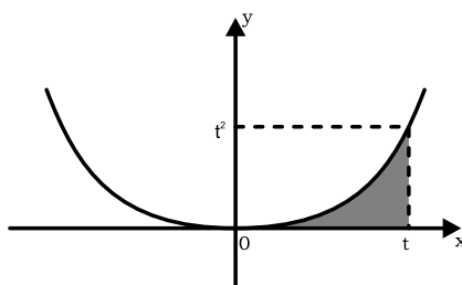
Figura 35: Área abaixo da curva
