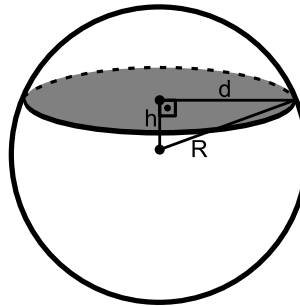
Figura 22: Área da secção
