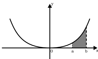
Figura 38: Área abaixo da curva no intervalo [a, b]
