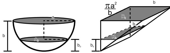
Figura 34: Volume da calota parabólica
