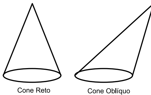
Figura 16: Tipos de cones
