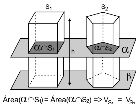
Figura 3: Ilustração do Princípio de Cavalieri
