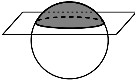
Figura 28: Calota esférica
