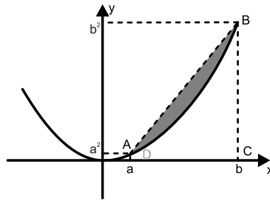
Figura 39: Área do segmento da Parábola
