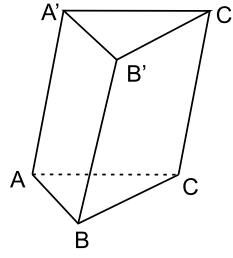
Figura 12: Prisma
