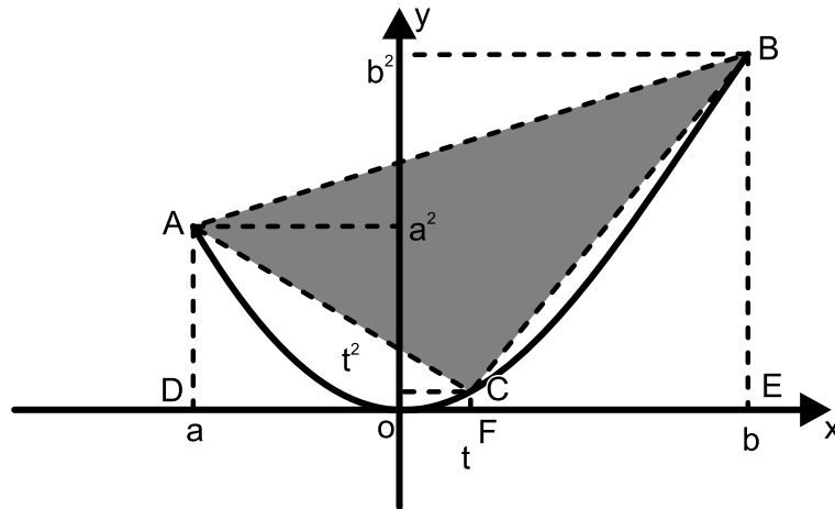
Figura 40: Maior triângulo inscrito
