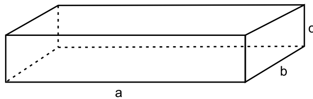
Figura 2: Paralelepípedo
