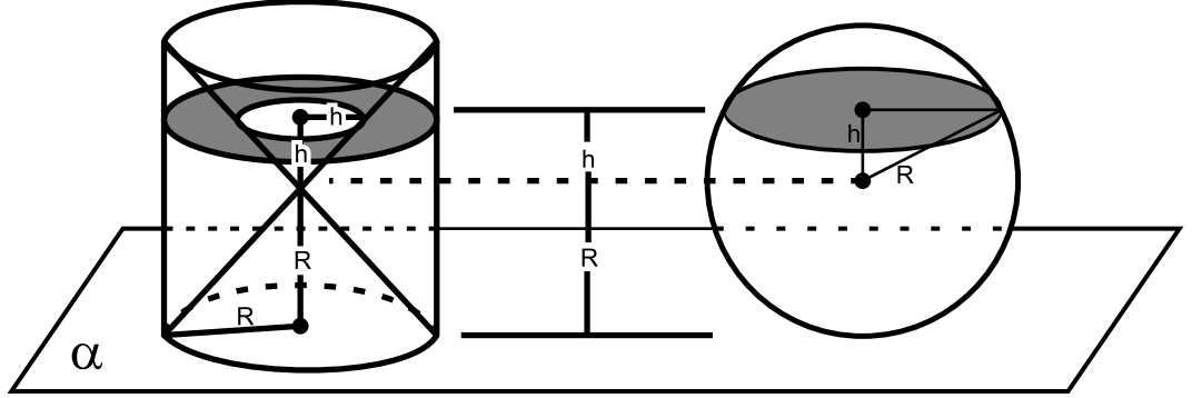
Figura 23: Volume da esfera
