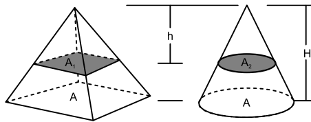
Figura 18: Volume do cone
