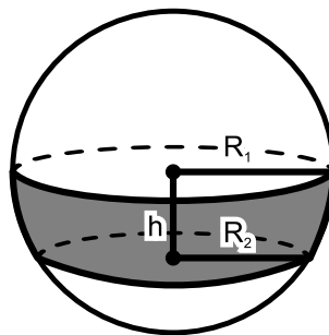
Figura 26: Segmento esférico
