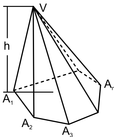
Figura 8: Pirâmide qualquer
