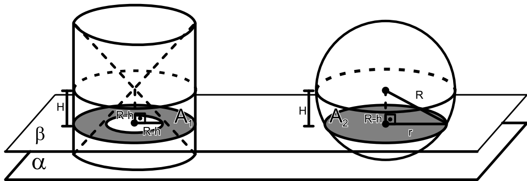
Figura 27: Volume do segmento esférico
