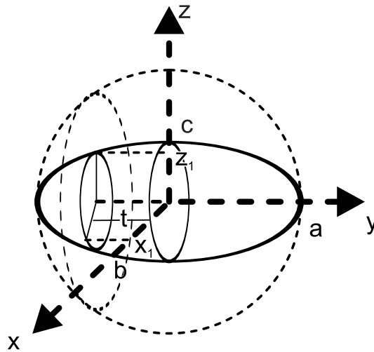
Figura 32: Elipsóide e Esfera
