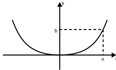
Figura 33: Parábola
