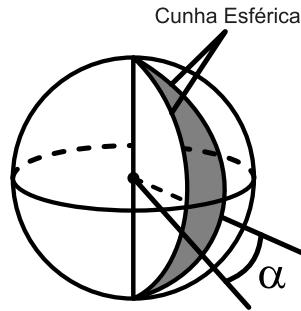
Figura 25: Cunha esférica
