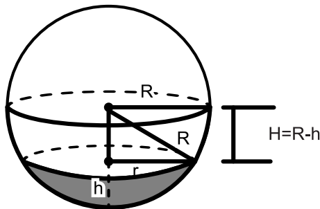
Figura 29: Volume da calota esférica
