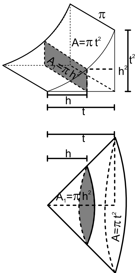
Figura 37: Comparando os sólidos
