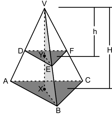
Figura 10: Razão de Semelhança
