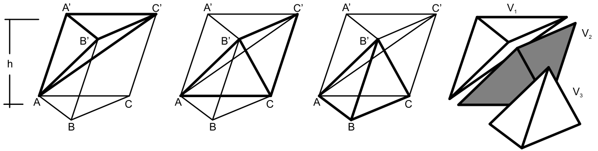
Figura 13: Partição do prisma em pirâmides
