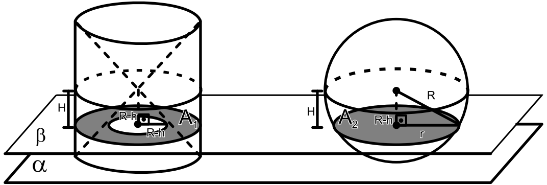
Figura 30: Equivalência entre as áreas
