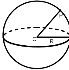
Figura 21: Esfera
