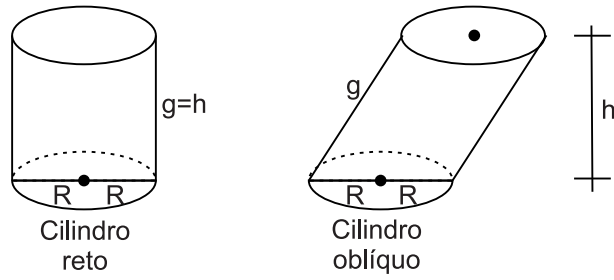
Figura 6: Cilindros
