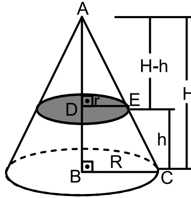
Figura 20: Tronco de cone
