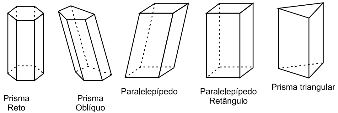
Figura 4: Prismas
