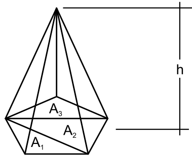
Figura 14: Volume de uma pirâmide qualquer
