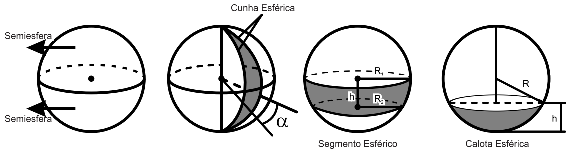
Figura 24: Partes da esfera
