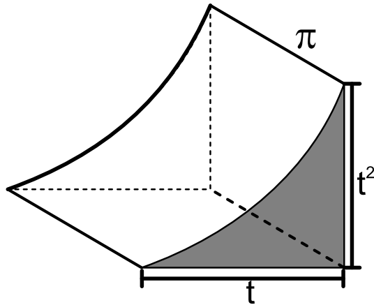
Figura 36: Sólido de altura \pi
