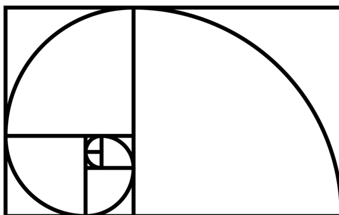
Figura 23 – A Espiral de Fibonacci
