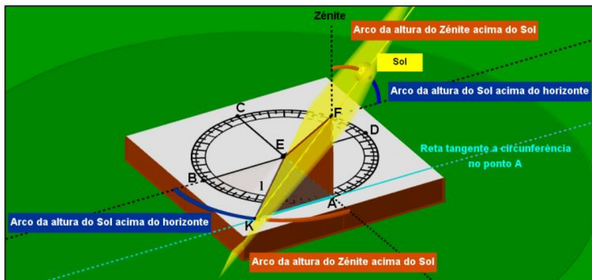
Figura 2 - Representação de uso do instrumento jacente no plano
