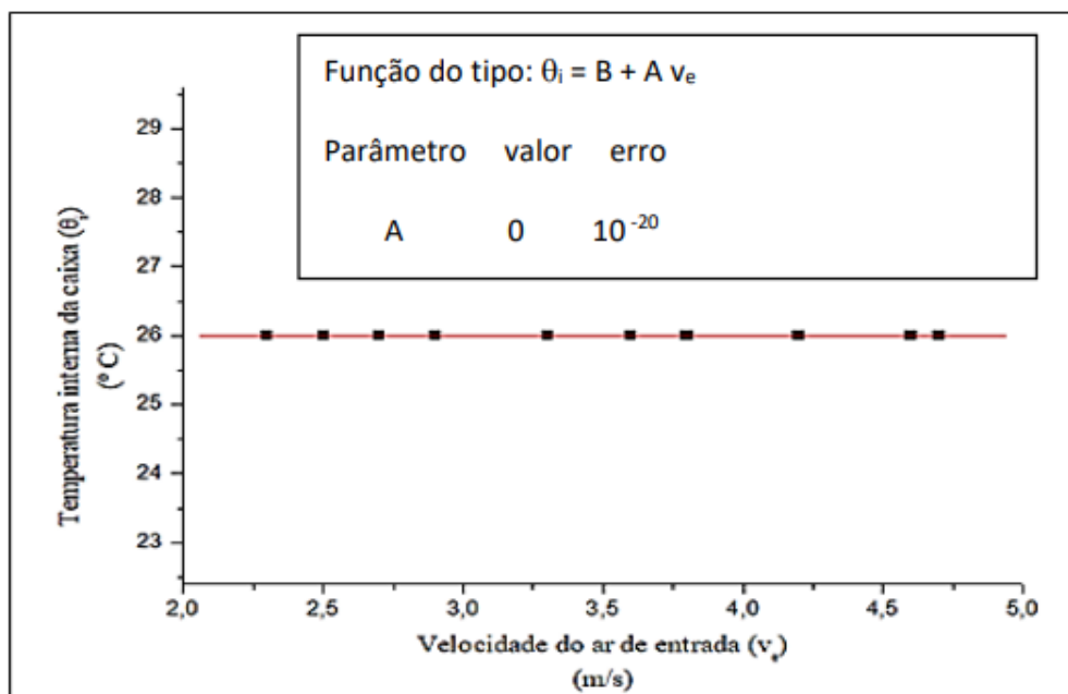
Figura 1 - Gráfico da temperatura interna ( \theta_i ) versus velocidade do ar de entrada ( v_e ) e a relação funcional entre as grandezas
