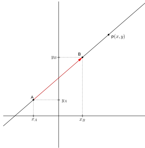
Figura 9: Reta \overline{AB}
