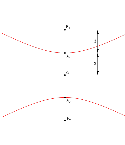
Figura 29: Exemplo 3.2.
