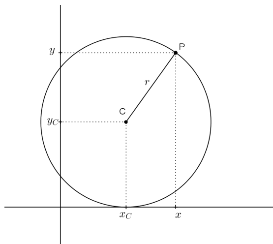
Figura 10: Circunferência
