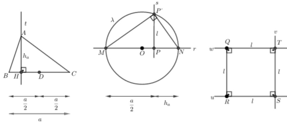
Figura 2.4: Triângulo enquadrável
