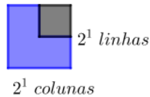
Figura 2.10: Tabuleiro 2^1 \times 2^1
