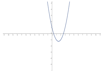
(b) b < 0
