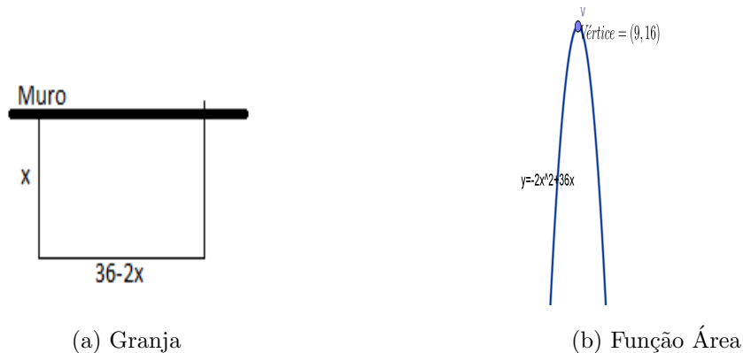
Figura 32: Granja e Função Área
