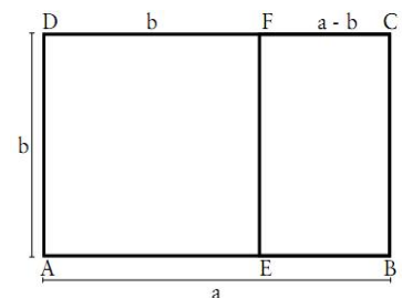
(b) Retângulo Áureo
