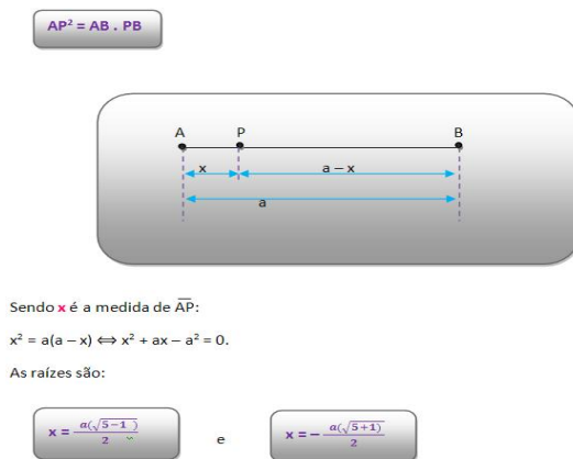
(a) Razão Áurea
