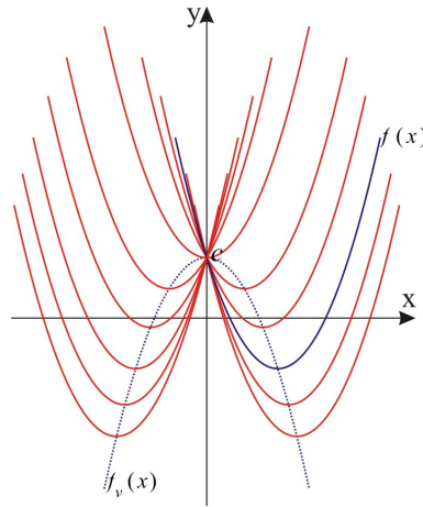
Figura 28: Movimento parabólico de uma parábola.
