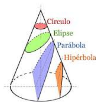
Figura 4: Seções Cônicas
