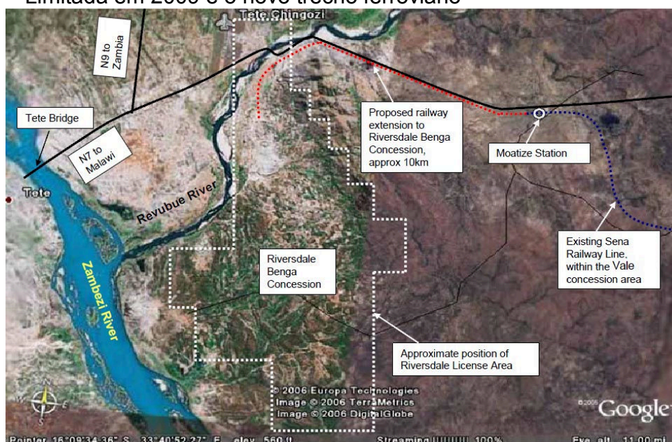
Figura 7 - Traçado da área de concessão da Riversdale Moçambique Limitada em 2009 e o novo trecho ferroviário
