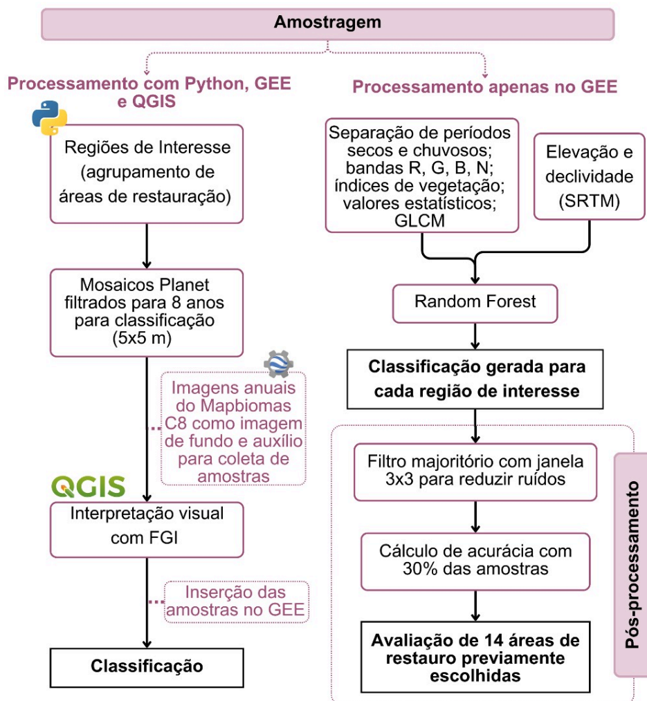
Figura 13 - Fluxograma da metodologia desenvolvida no estudo.
