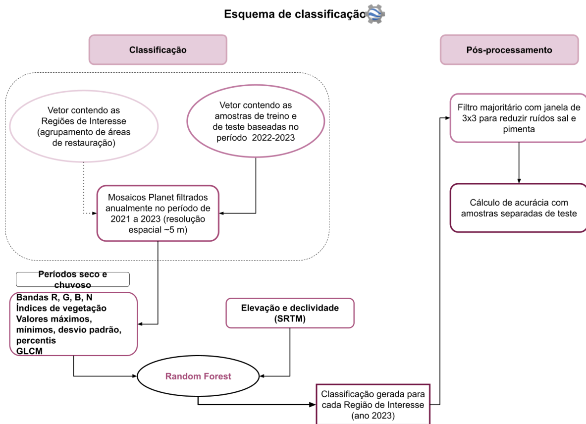
Figura 6 - Demonstração dos passos executados na classificação supervisionada.
