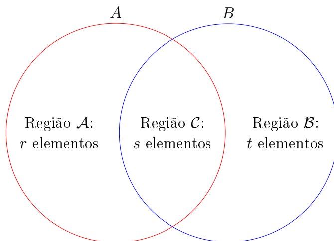
Figura 24: Diagrama dos Conjuntos A e B.
