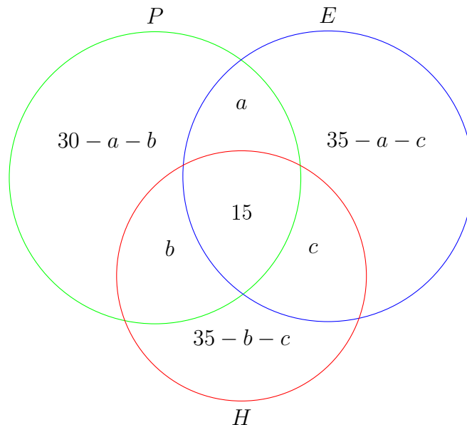
Figura 20: Diagrama dos Conjuntos P, E e H.
