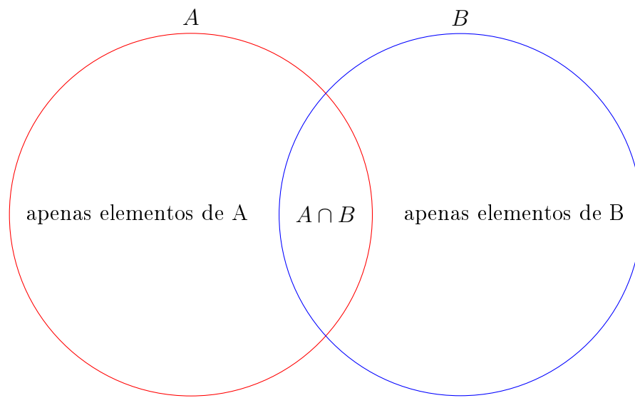
Figura 25: Diagrama dos Conjuntos A e B.
