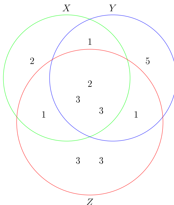
Figura 27: Diagrama dos Conjuntos X, Y e Z.
