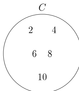
Figura 14: Representação do Conjunto C.
