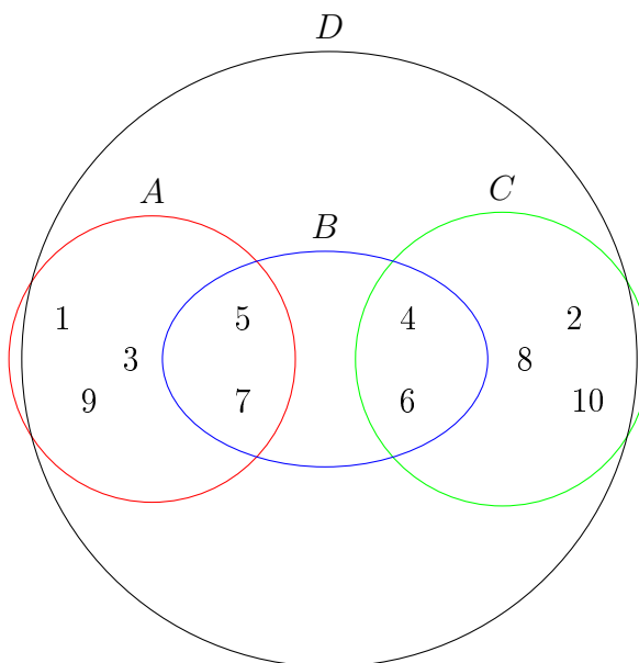
Figura 19: Representação dos Conjuntos A , B , C e D .
