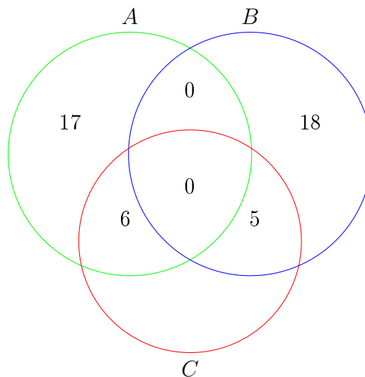
Figura 36: Representação do Diagrama dos Conjuntos A, B e C.
