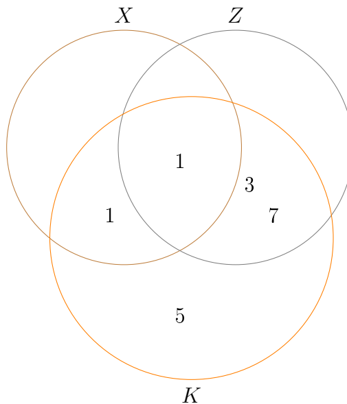
Figura 29: Diagrama dos Conjuntos X , Z e K .
