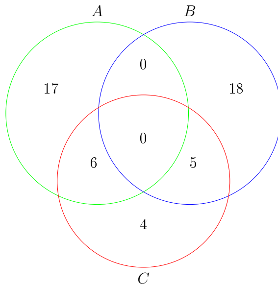
Figura 37: Representação do Diagrama dos Conjuntos A, B e C.
