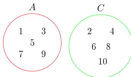
Figura 17: Representação dos Conjuntos A e C.
