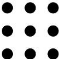
Figura 3: Representação do Número 9 em Forma Geométrica.
