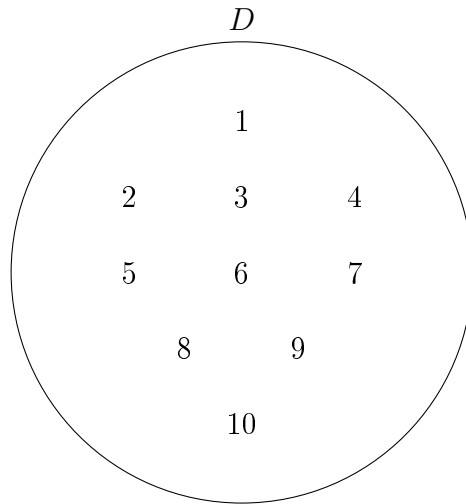
Figura 15: Representação do Conjunto D .
