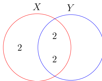
Figura 32: Diagrama dos Conjuntos X e Y.
