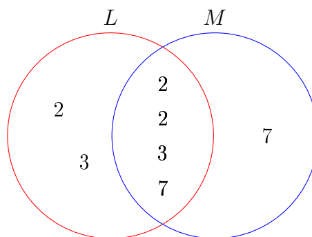
Figura 22: Diagrama dos Conjuntos L e M.
