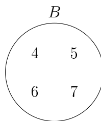
Figura 13: Representação do Conjunto B.
