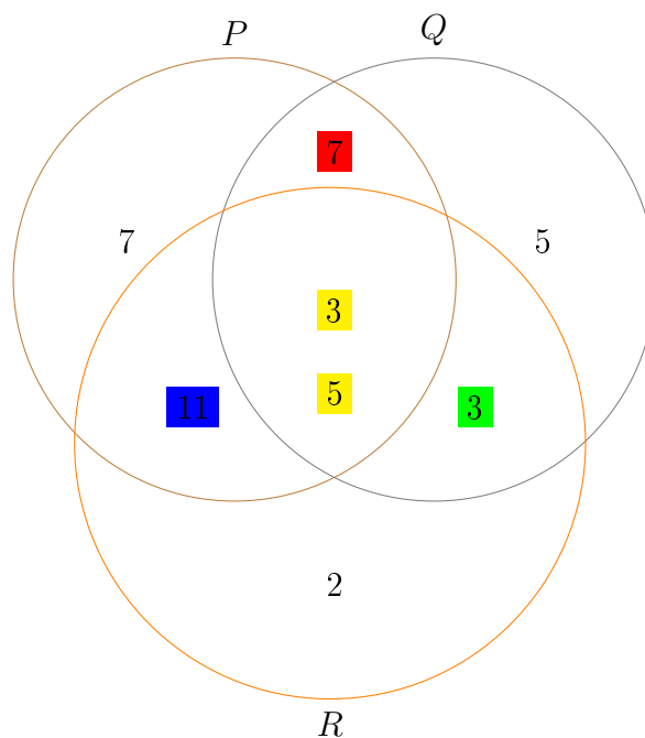
Figura 23: Diagrama dos Conjuntos P, Q e R.
