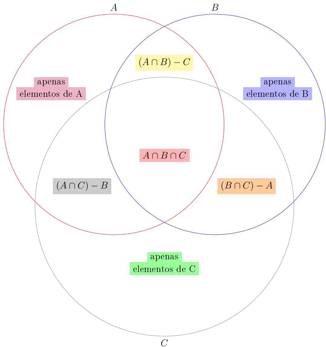
Figura 26: Diagrama dos Conjuntos A, B e C.
