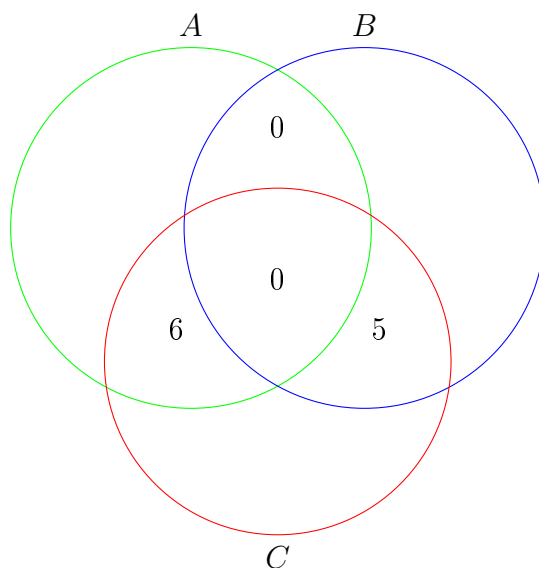
Figura 34: Representação do Diagrama dos Conjuntos A , B e C .
