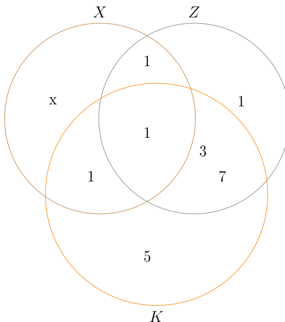
Figura 31: Diagrama dos Conjuntos X, Z e K.
