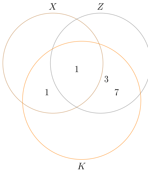
Figura 28: Diagrama dos Conjuntos X , Z e K .
