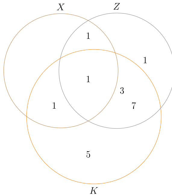
Figura 30: Diagrama dos Conjuntos X , Z e K .
