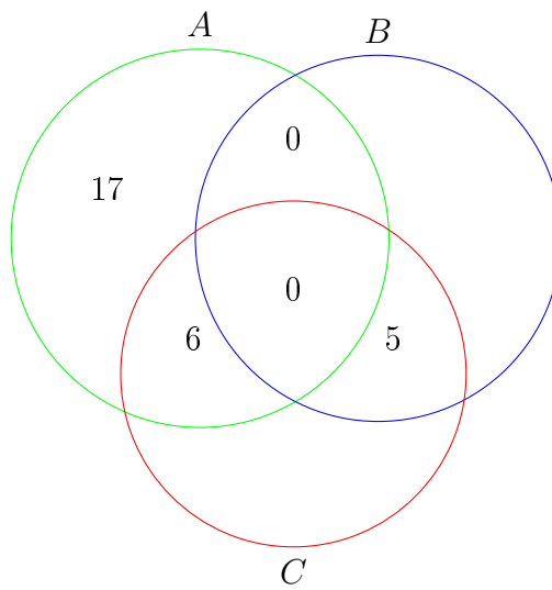
Figura 35: Representação do Diagrama dos Conjuntos A, B e C.
