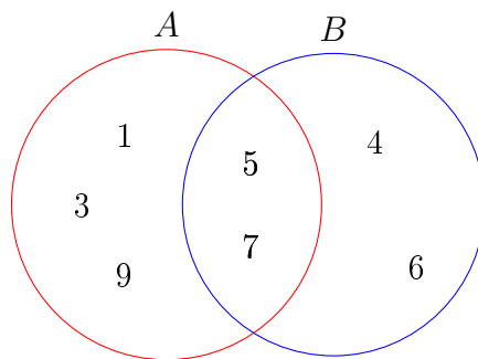
Figura 16: Representação dos Conjuntos A e B.
