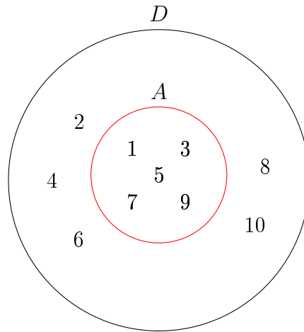
Figura 18: Representação dos Conjuntos A e D.
