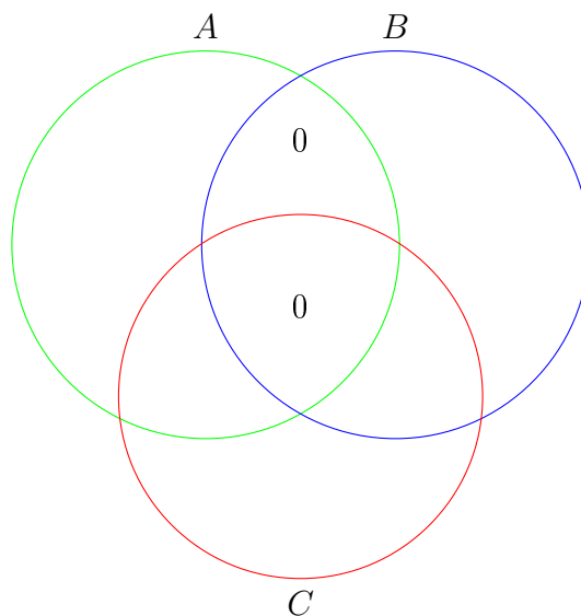
Figura 33: Representação do Diagrama dos Conjuntos A , B e C .
