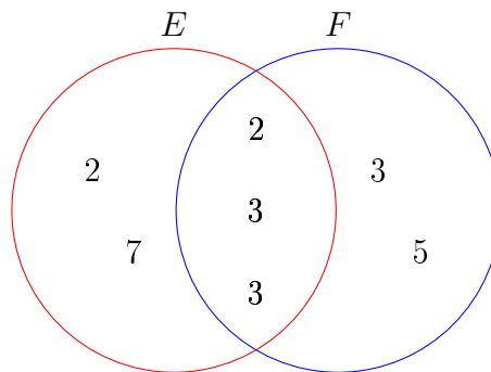
Figura 21: Diagrama dos Conjuntos E e F.
