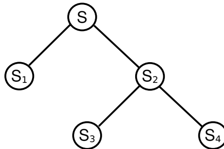
Figura 2.1: Árvore Branch-and-Bound , de subproblemas.
