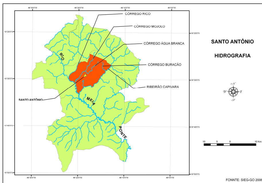
Figura 8: Hidrografia do município de Santo Antônio de Goiás.
