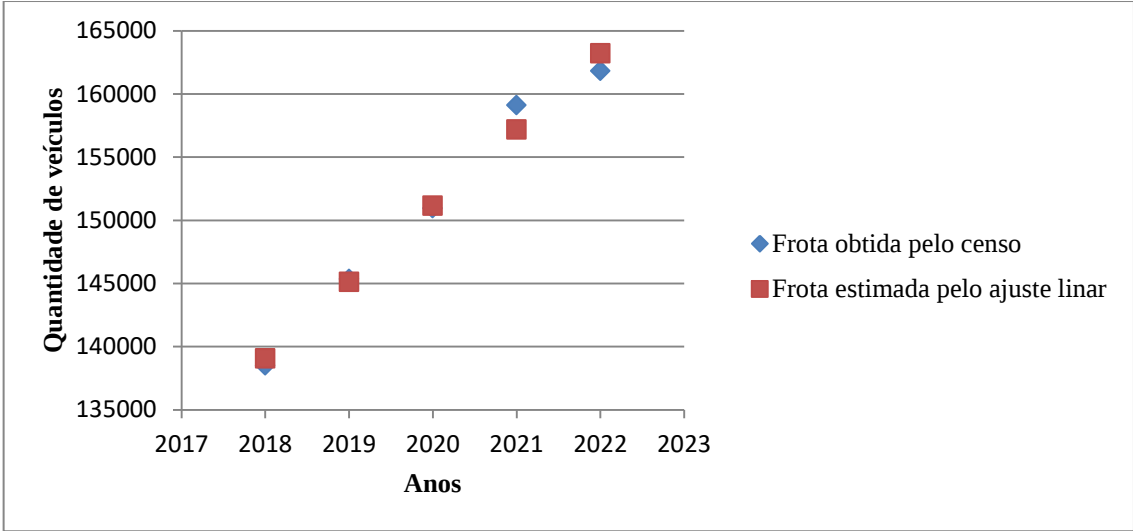
Gráfico 1 — Frota de veículos em Aparecida de Goiânia
