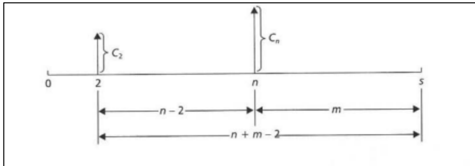
Figura 6 — Representação dos valores nominais e das datas focais
