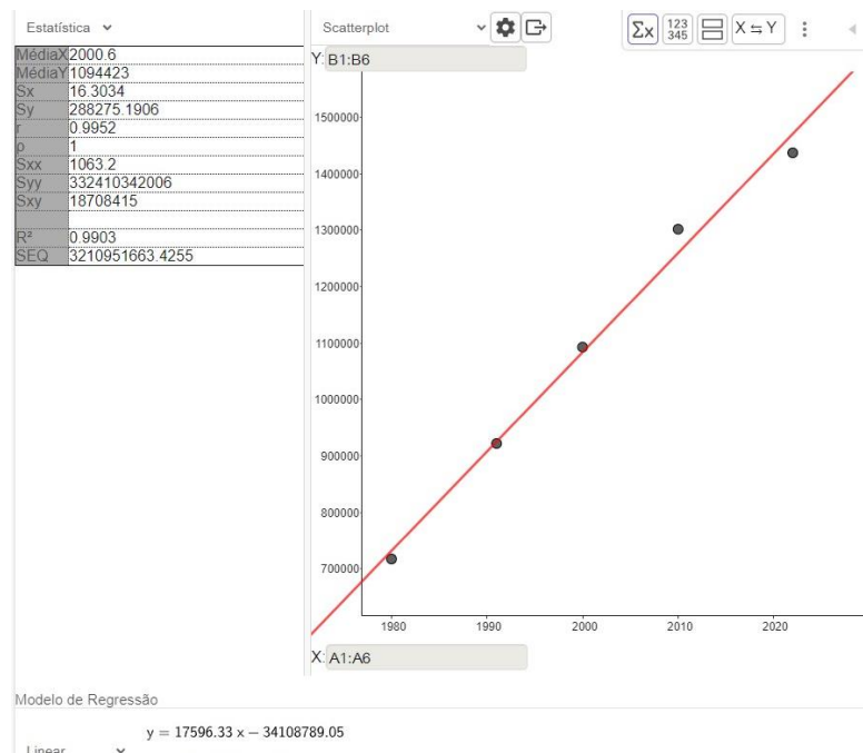
Figura 3 — Ajuste linear da população em Goiânia entre 1980 e 2022 realizado no Geogebra
