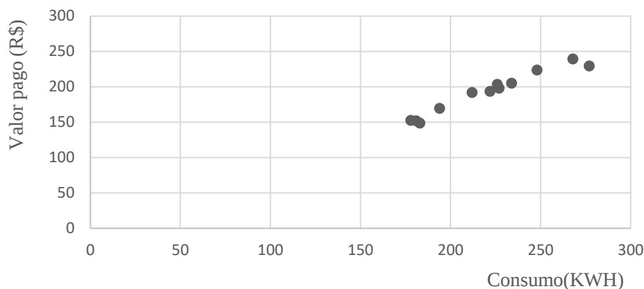
Gráfico 3 — Gráfico de dispersão que relaciona o consumo e o valor pago na conta de energia elétrica
