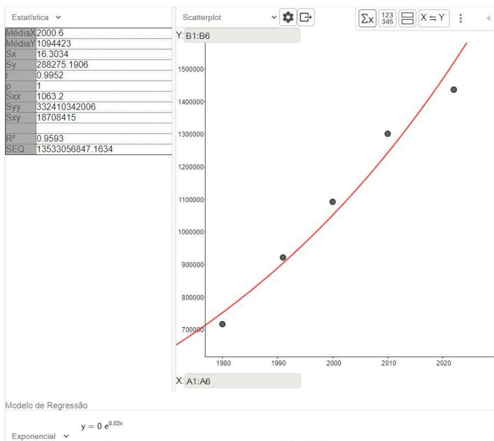
Figura 5 — Ajuste exponencial da população em Goiânia entre 1980 e 2022 feito no Geogebra
