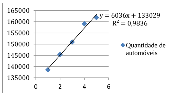
Gráfico 2 — Ajuste Linear da Frota de Veículos em Aparecida de Goiânia realizado no Excel
