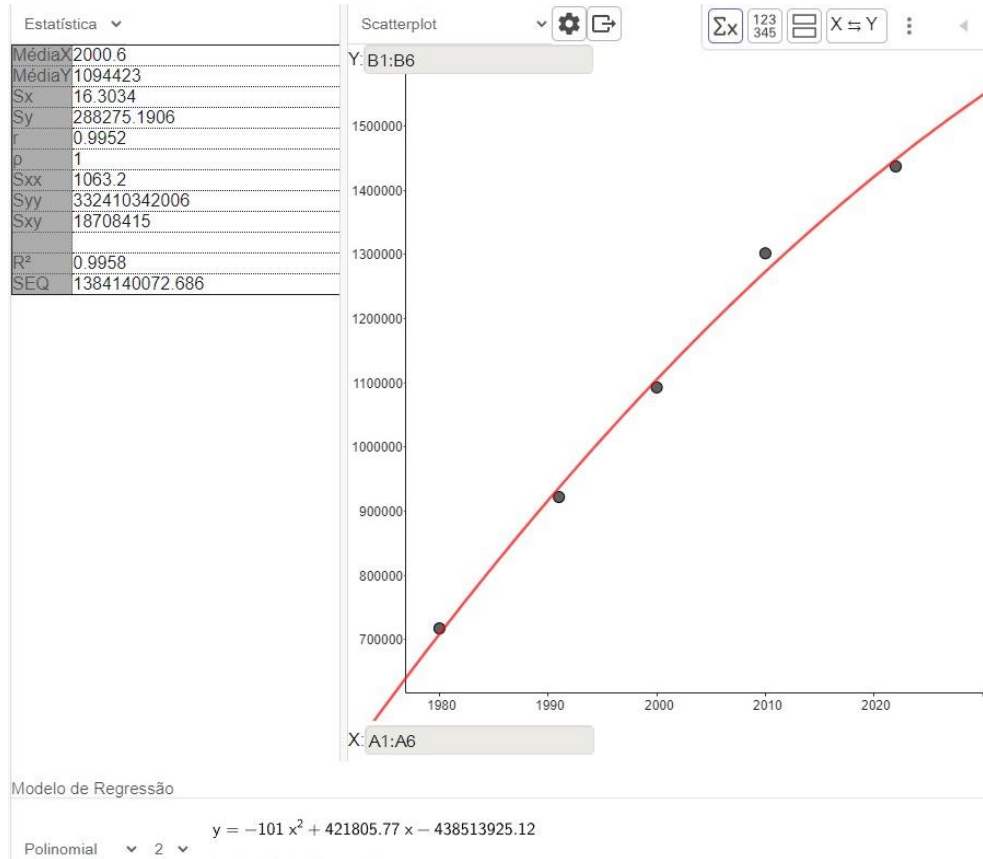
Figura 4 — Ajuste quadrático da população em Goiânia entre 1980 e 2022 feito no Geogebra
