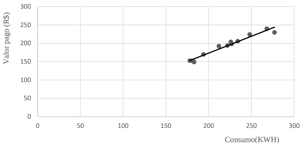
Gráfico 4 — Linha de tendência que relaciona o consumo e o valor pago na conta de energia elétrica
