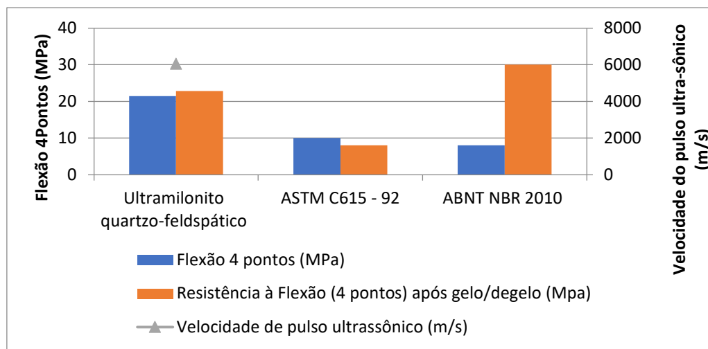
Gráfico 5: Resultados de resistência a flexão em 4 pontos (seco e após congelamento/degelo) obtidos para o Ultramilonito Quartzo Feldspático.
