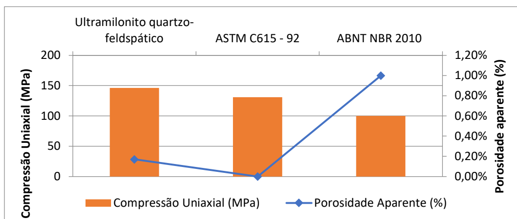
Gráfico 3: Resultados de resistência a compressão uniaxial obtidos para o Ultramilonito Quartzo Feldspático.
