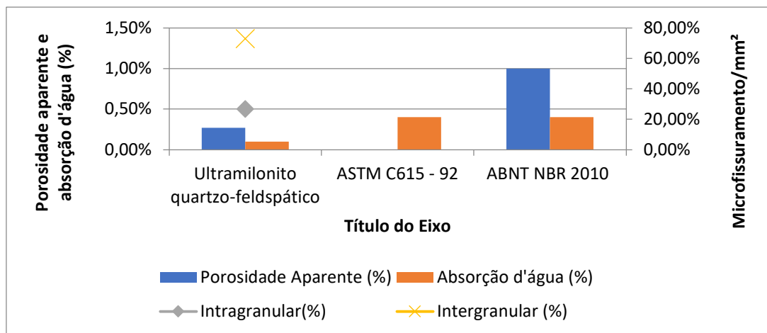
Gráfico 2: Resultados de porosidade aparente e absorção d'água para o Ultramilonito Quartzo Feldspático.
