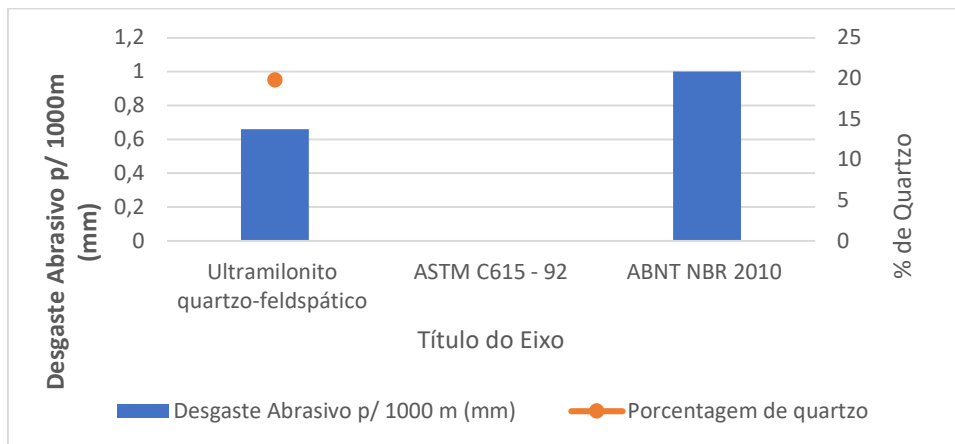
Gráfico 6: Resultados de resistência ao desgaste abrasivo obtidos para o Ultramilonito, relacionados com a porcentagem de quartzo.
