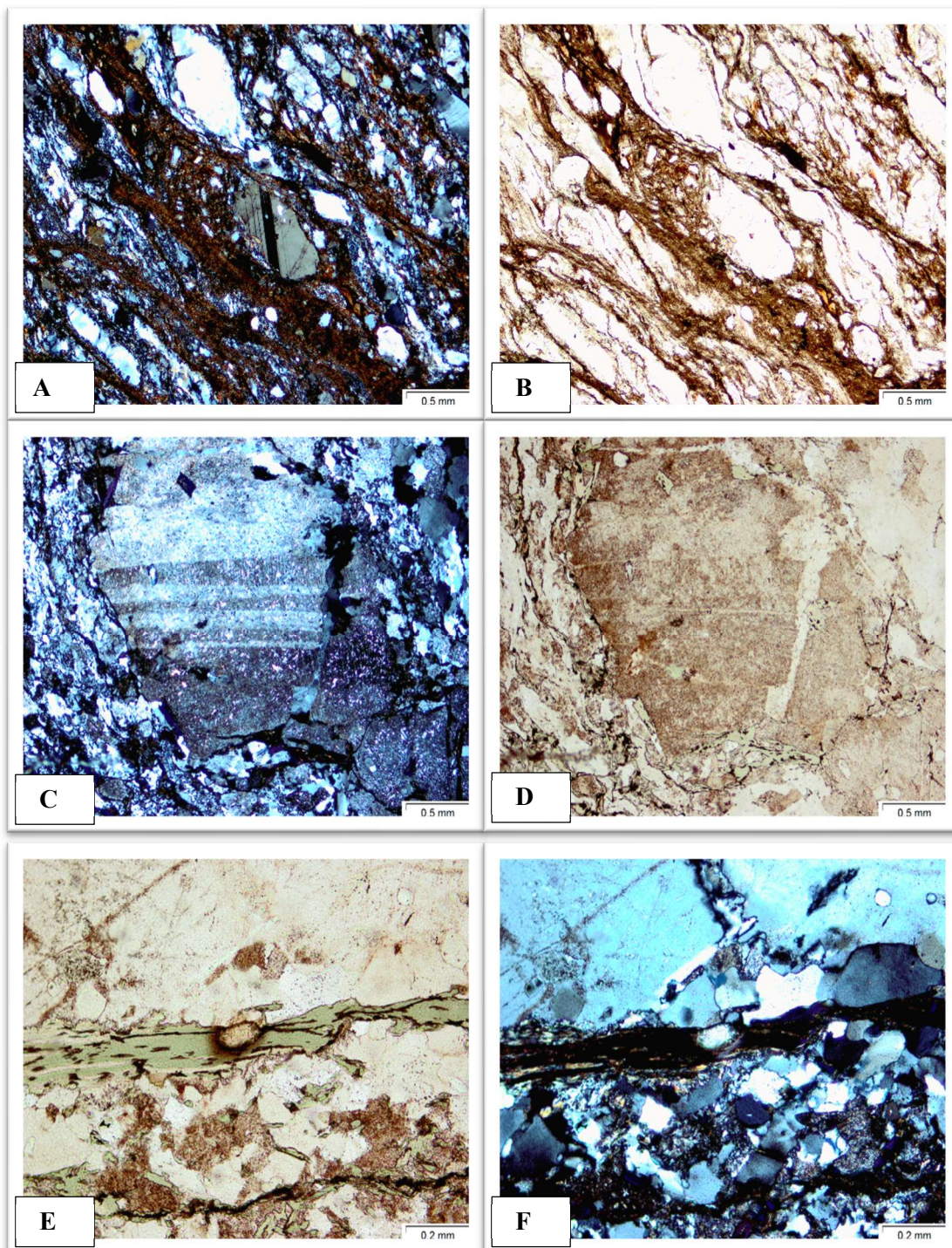
Figura 4 – (A) Matriz da rocha, dando destaque a cristais de plagioclásio, alguns rotacionados e aos óxidos e hidróxidos de ferro preenchendo as microfissuras na luz ortoscópica; (B) Matriz da rocha, dando destaque a cristais de plagioclásio, alguns rotacionados e aos óxidos e hidróxidos de ferro preenchendo as microfissuras na luz natural; (C) Plagioclásio sautirizado com inclusões de clorita na luz ortoscópica; (D) Plagioclásio sautirizado com inclusões de clorita na luz natural; (E) Zircão incluído no cristal de clorita na luz ortoscópica; (F) Zircão incluído no cristal de clorita na luz natural.
